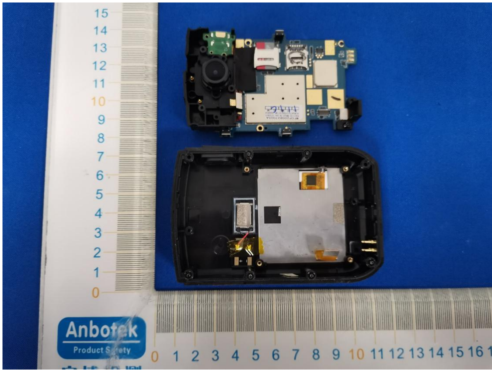
BT&WIFI ANT
