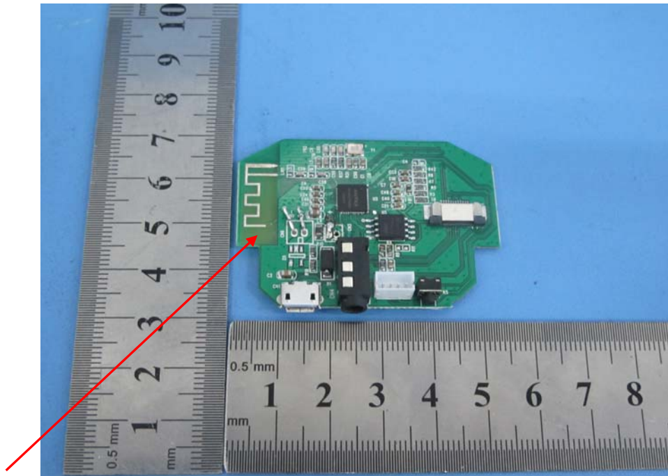
2.4G Antenna
