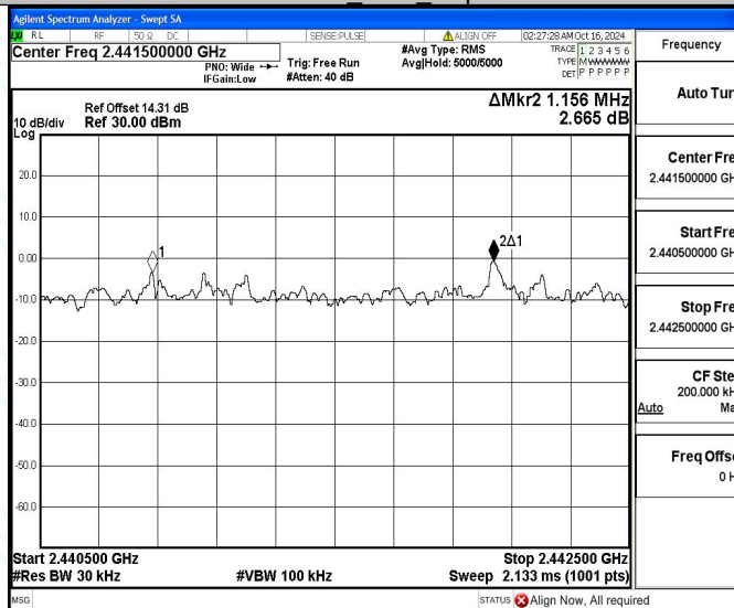
3DH5_Ant1_Hop
