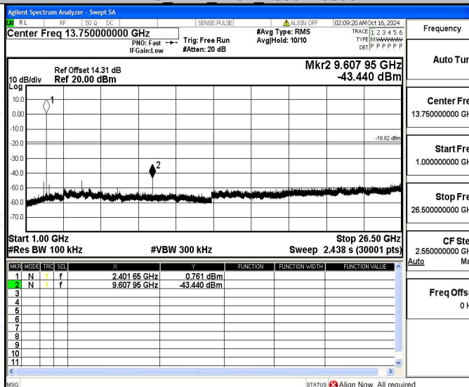
DH5_Ant1_2402_1000~26500
