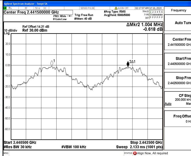
2DH5_Ant1_Hop
