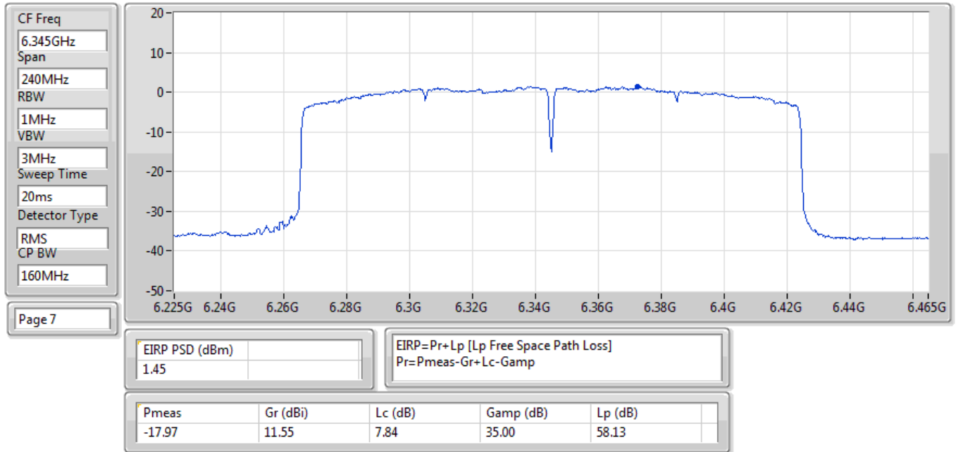
EIRP PSD;Band:6.2G;ax160,BF;BWch:160MHz;Nss:1,(M0);Nant:2;Ch:6345MHz;TX
