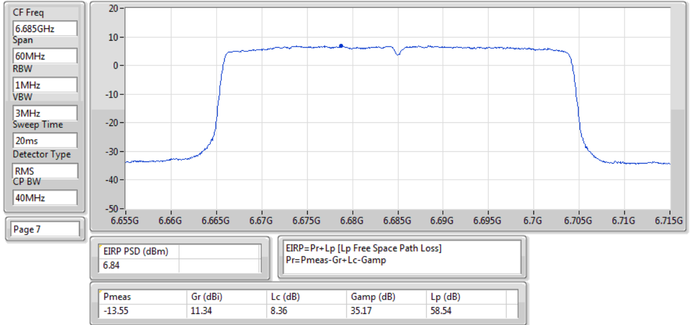
EIRP PSD;Band:6.7G;ax40,BF;BWch:40MHz;Nss:1,(M0);Nant:2;Ch:6685MHz;TX
