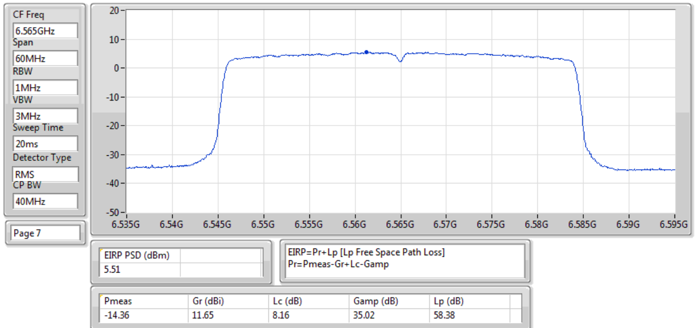
EIRP PSD;Band:6.7G;ax40,BF;BWch:40MHz;Nss:1,(M0);Nant:2;Ch:6565MHz;TX
