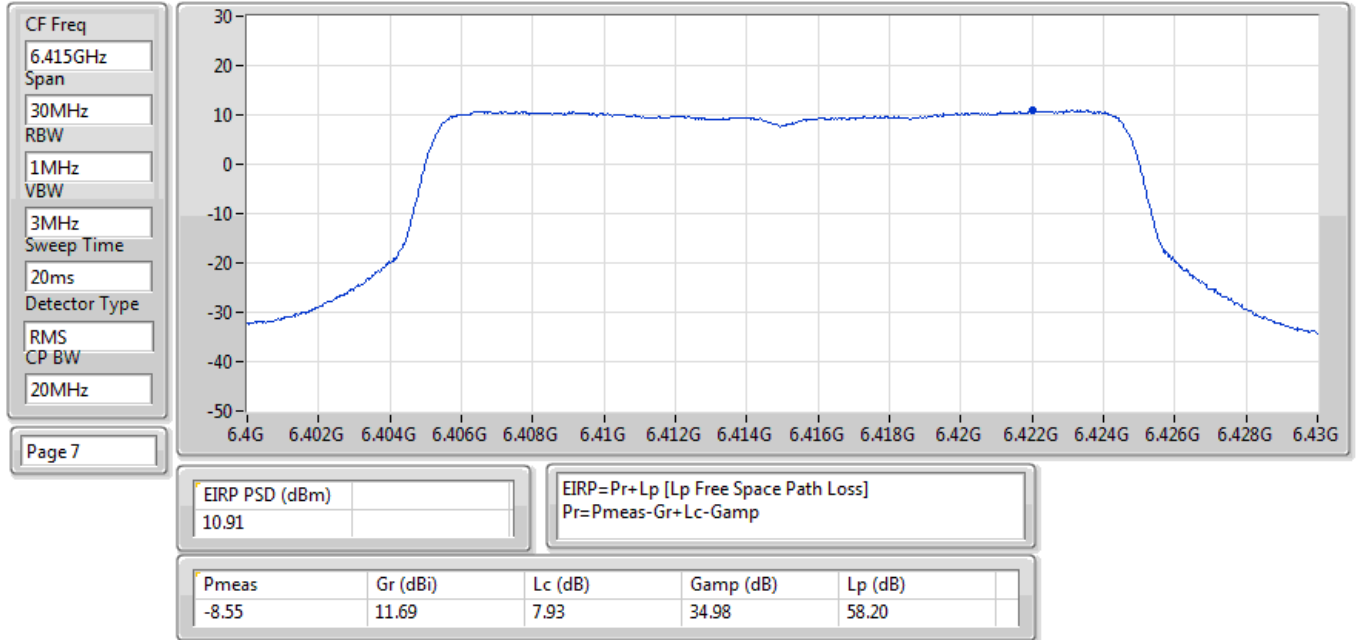
EIRP PSD;Band:6.2G;ax20,BF;BWch:20MHz;Nss:1,(M0);Nant:2;Ch:6415MHz;TX
