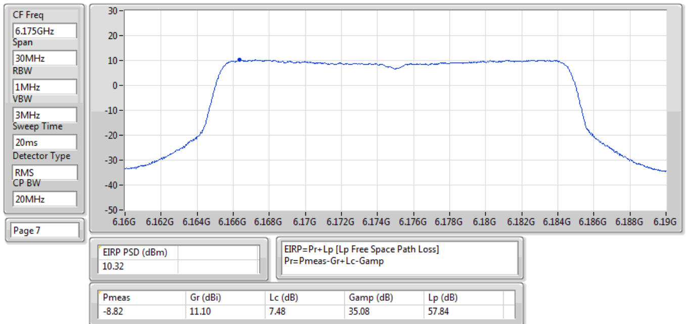
EIRP PSD;Band:6.2G;ax20,BF;BWch:20MHz;Nss:1,(M0);Nant:2;Ch:6175MHz;TX
