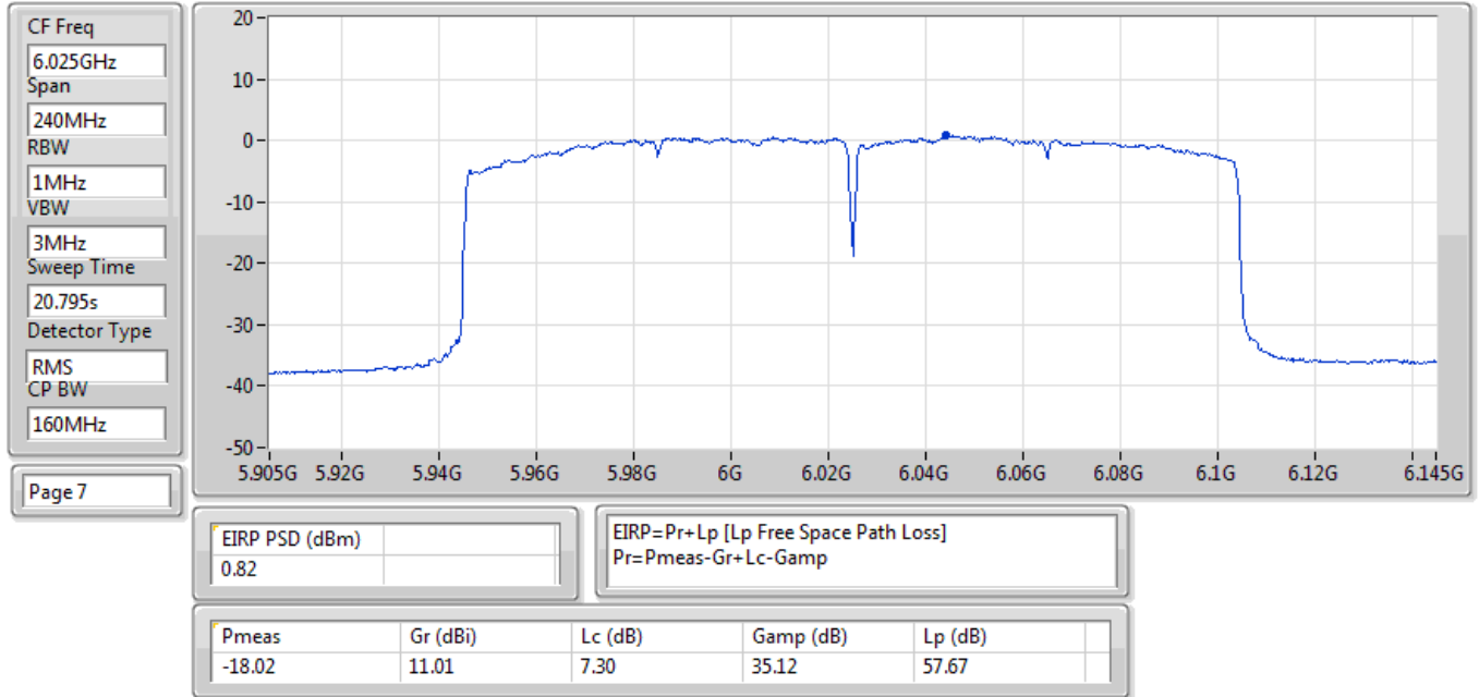
EIRP PSD;Band:6.2G;ax160,BF;BWch:160MHz;Nss:1,(M0);Nant:2;Ch:6025MHz;TX
