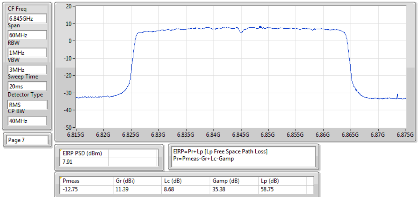
EIRP PSD;Band:6.7G;ax40,BF;BWch:40MHz;Nss:1,(M0);Nant:2;Ch:6845MHz;TX
