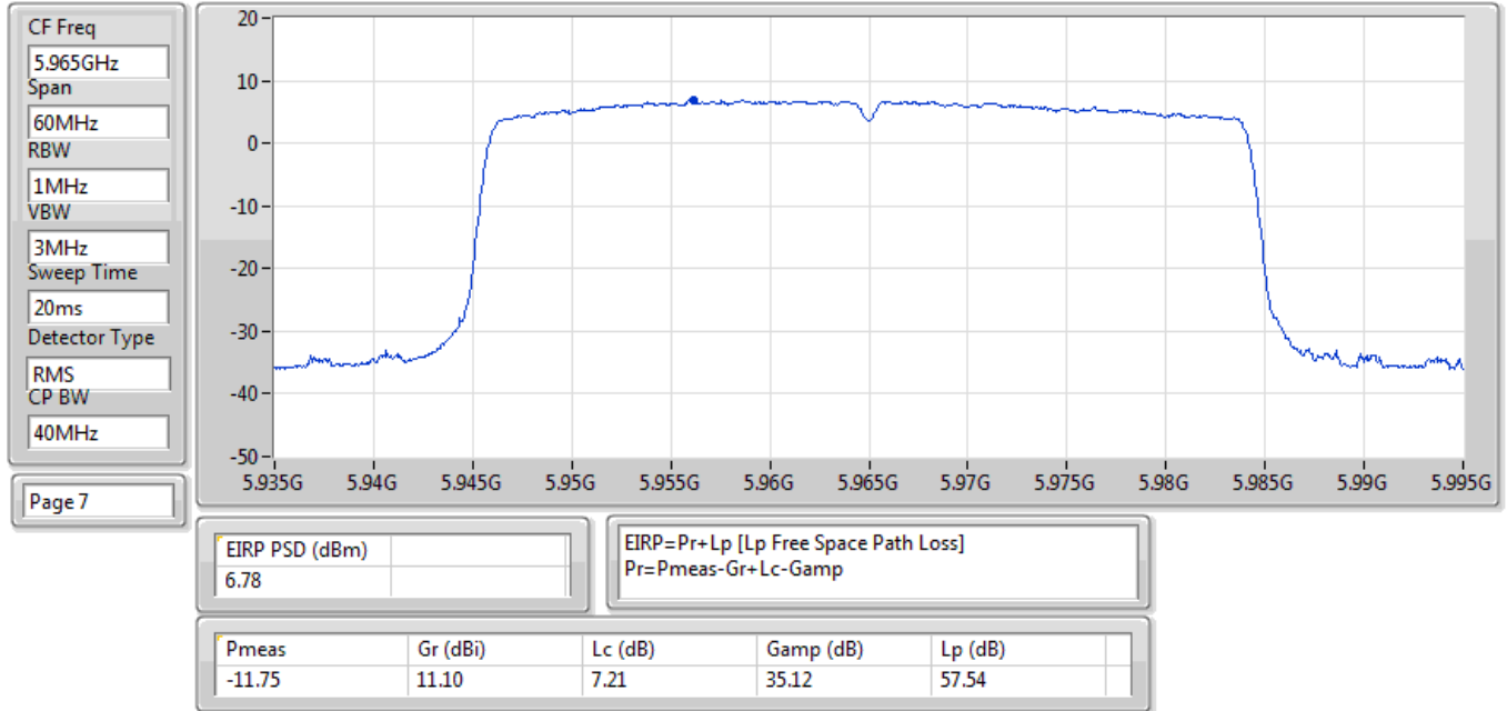
EIRP PSD;Band:6.2G;ax40,BF;BWch:40MHz;Nss:1,(M0);Nant:2;Ch:5965MHz;TX
