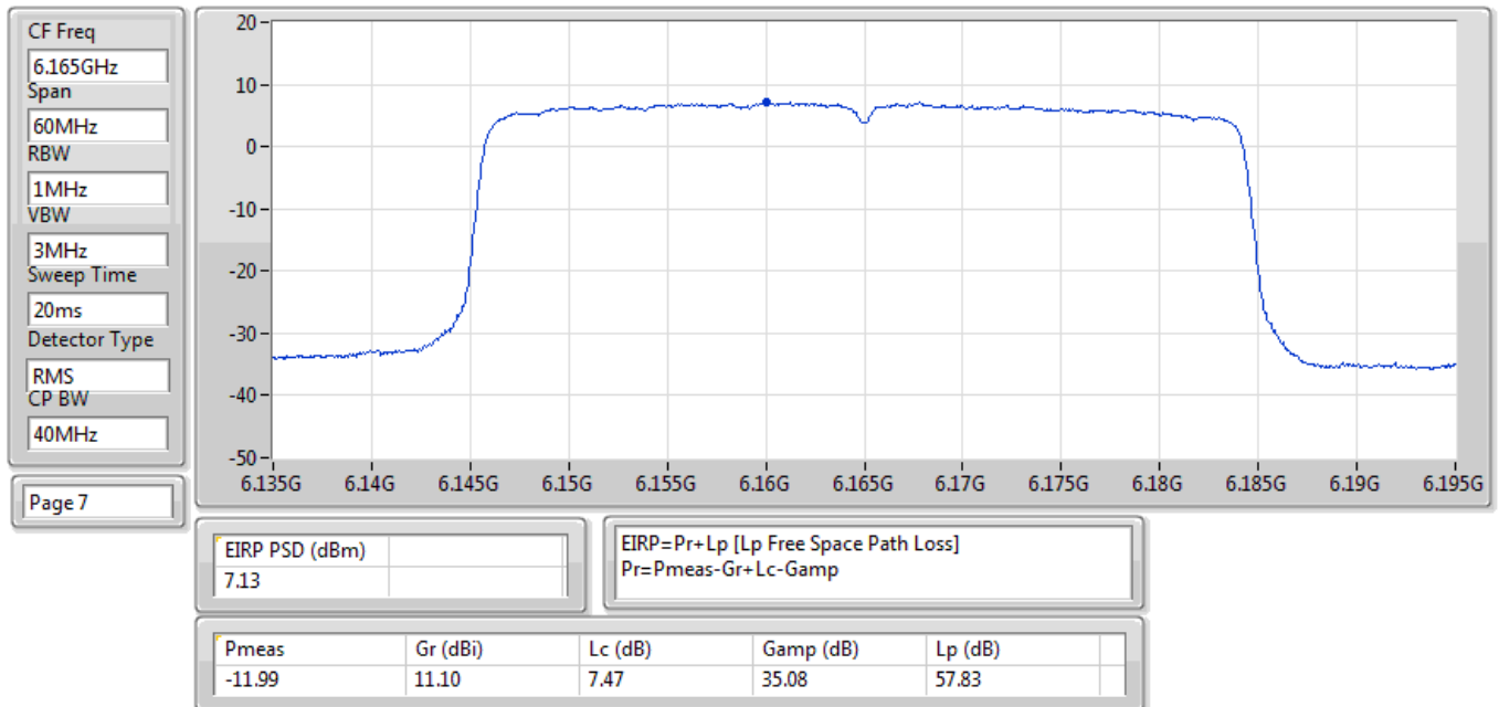
EIRP PSD;Band:6.2G;ax40,BF;BWch:40MHz;Nss:1,(M0);Nant:2;Ch:6165MHz;TX
