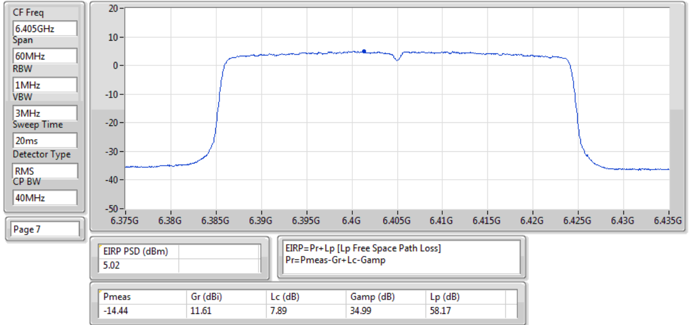
EIRP PSD;Band:6.2G;ax40,BF;BWch:40MHz;Nss:1,(M0);Nant:2;Ch:6405MHz;TX
