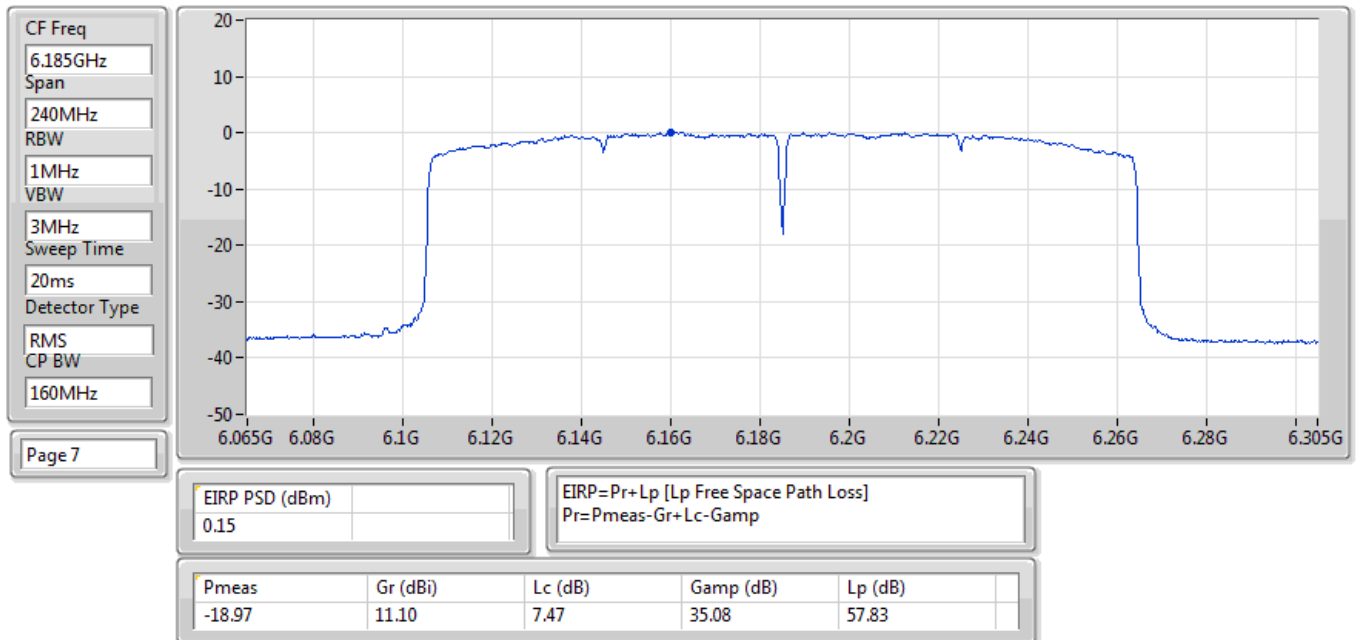
EIRP PSD;Band:6.2G;ax160,BF;BWch:160MHz;Nss:1,(M0);Nant:2;Ch:6185MHz;TX
