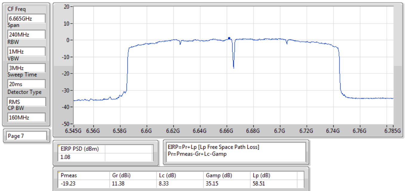
EIRP PSD;Band:6.7G;ax160,BF;BWch:160MHz;Nss:1,(M0);Nant:2;Ch:6665MHz;TX
