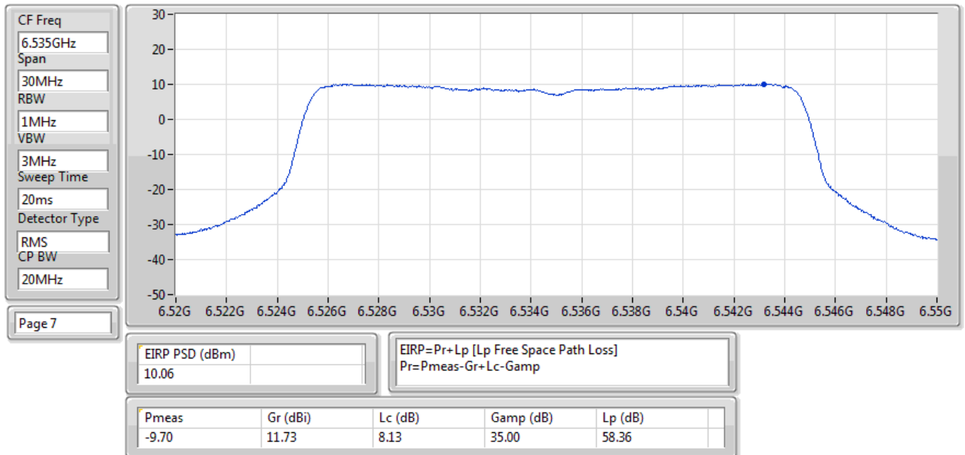
EIRP PSD;Band:6.7G;ax20,BF;BWch:20MHz;Nss:1,(M0);Nant:2;Ch:6535MHz;TX
