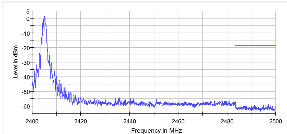
Screenshot: Upperband edge sweep
