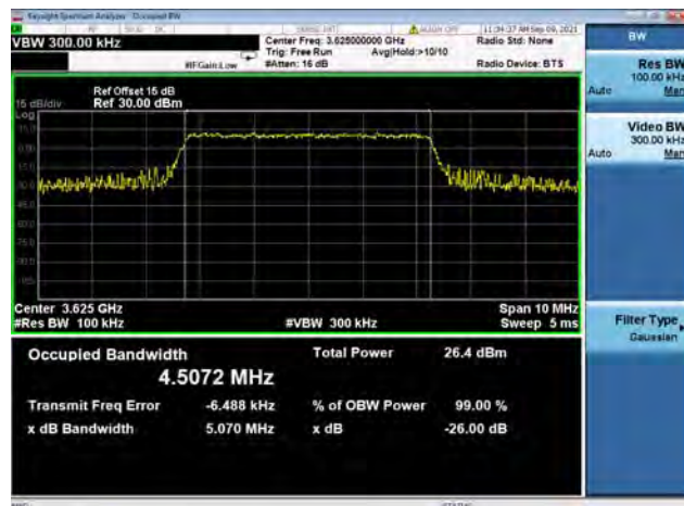
Band48 / 5MHz / Mid CH / 16QAM
