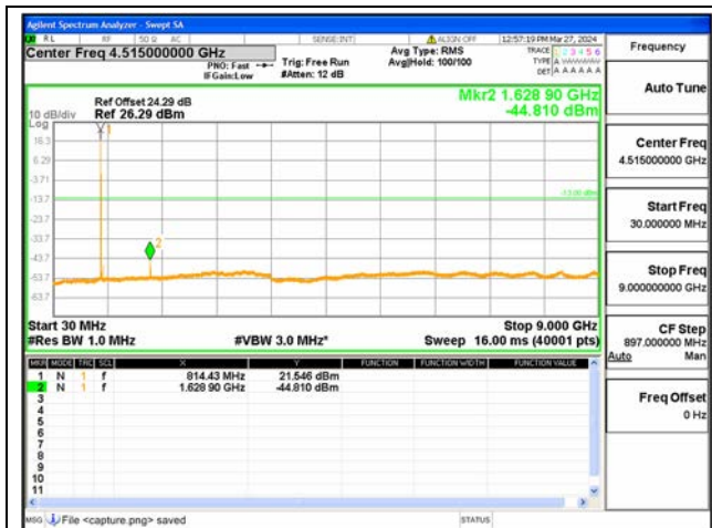
B26 Part90 / 5MHz / Low CH / QPSK
