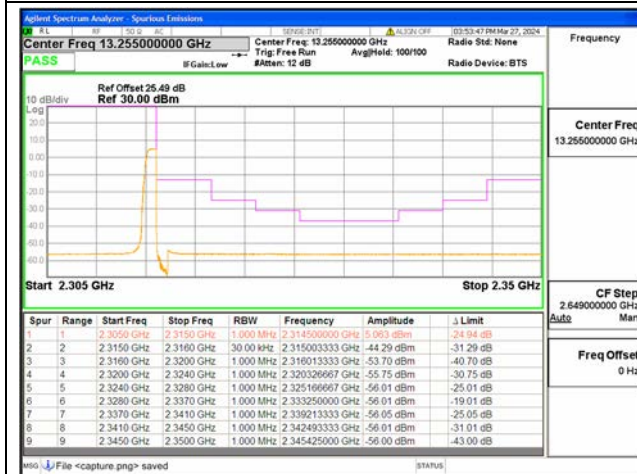
B30 / 5MHz / High CH / QPSK / 1 RB
