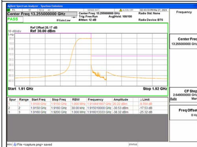
B25 / 5MHz / High CH / QPSK / 1 RB
