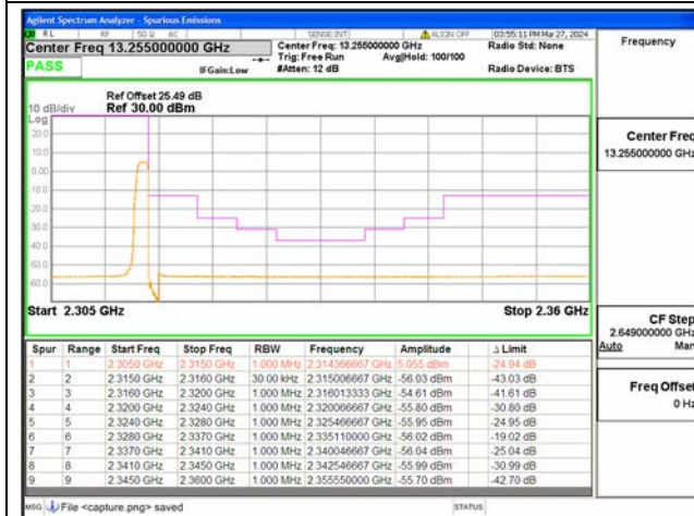
B30 / 10MHz / High CH / QPSK / 1 RB
