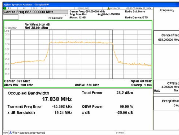
B71 / 20MHz / 64QAM / Mid CH
