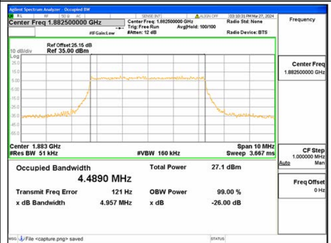
B25 / 5MHz / QPSK/ Mid CH
