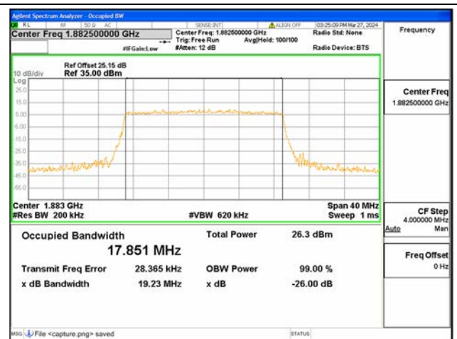
B25 / 20MHz / 16QAM / Mid CH
