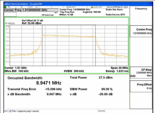
B25 / 10MHz / QPSK / High CH
