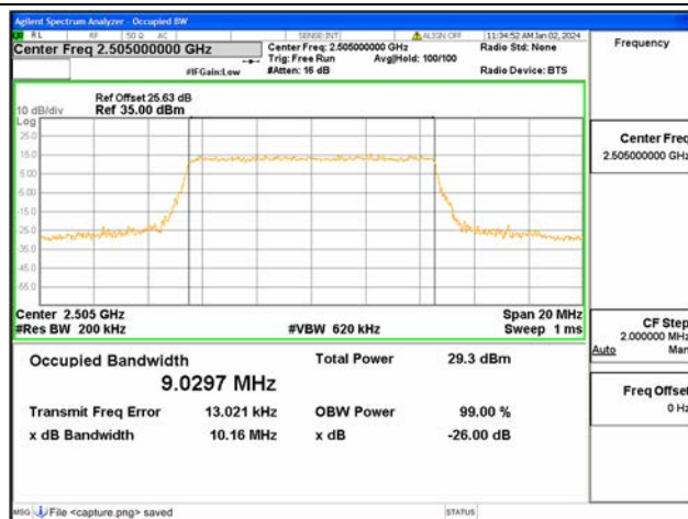
B7 / 10MHz / 64QAM/ Low CH
