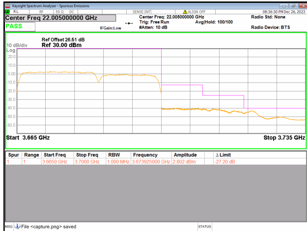
48C / 20+15MHz / High CH / QPSK / 100#0-75#0
