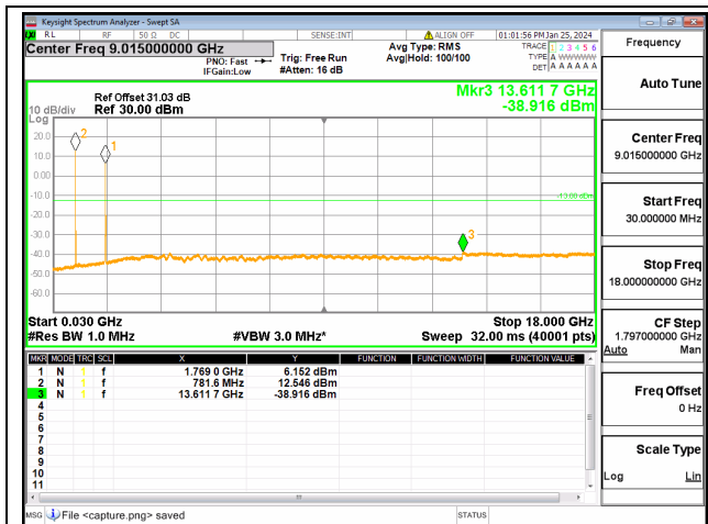
13A-66A / 10+20MHz / QPSK / Low+High CH / 50@0-100@0
