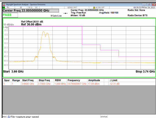
48C / 20+20MHz / High CH / QPSK / 1#99-1#0
