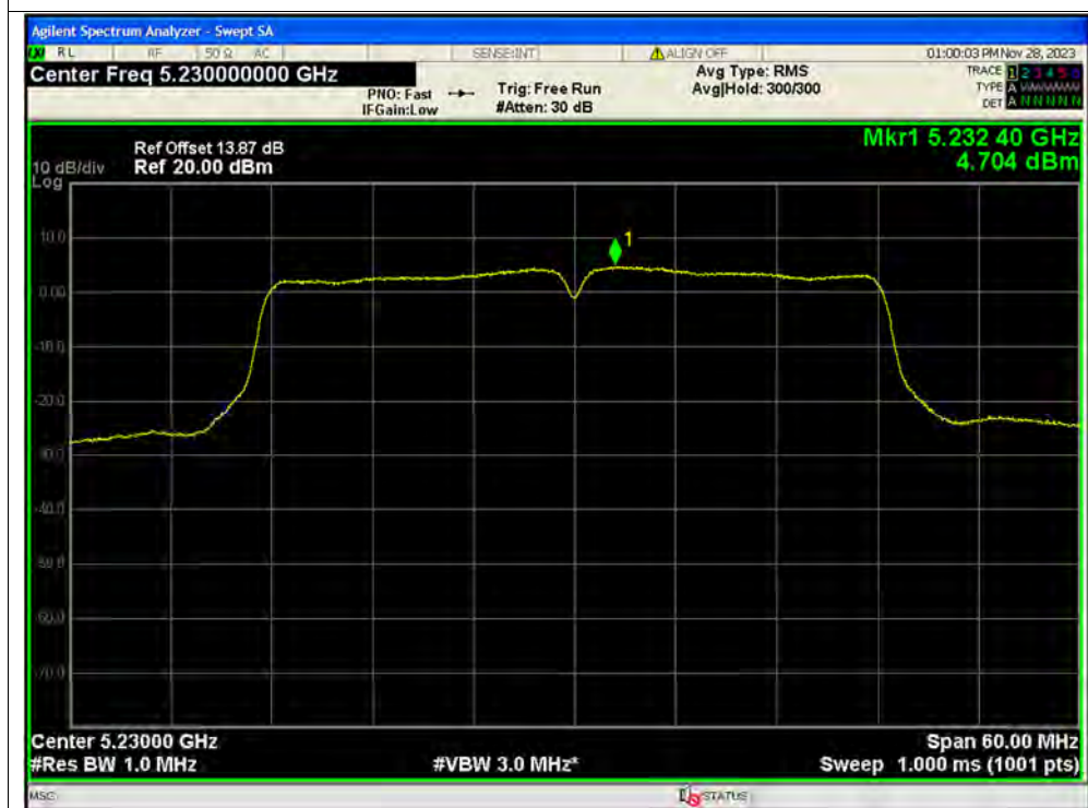
PSD NVNT n40 5230MHz Ant2 MIMO
