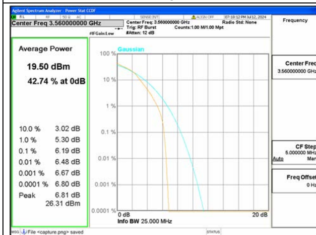
B48 / 20MHz / Low CH / 16QAM
