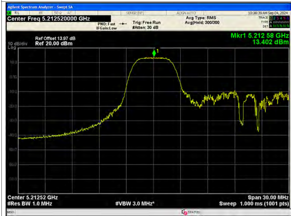
PSD NVNT ax20 52@37 5220MHz Ant2 MIMO
