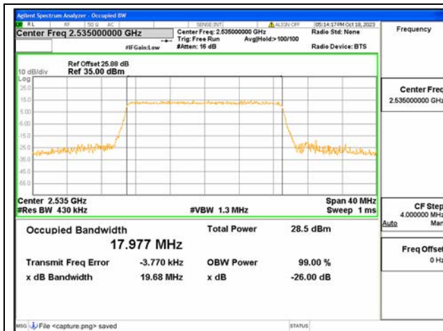
B7 / 20MHz / 64QAM/ Mid CH
