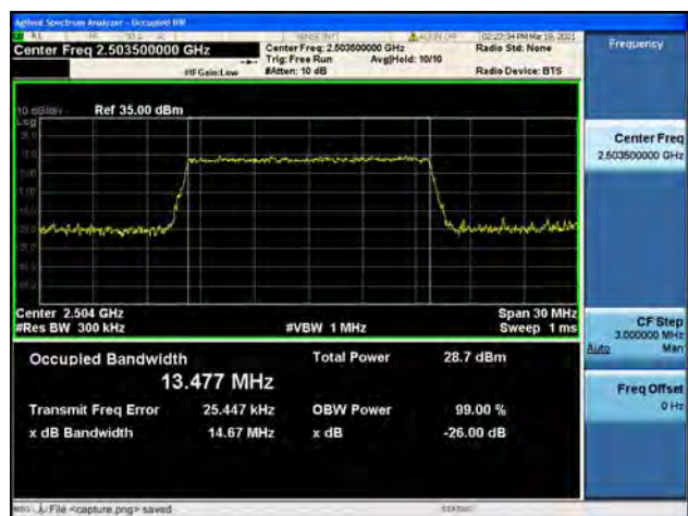
Band41 / 15MHz / Mid CH / QPSK
