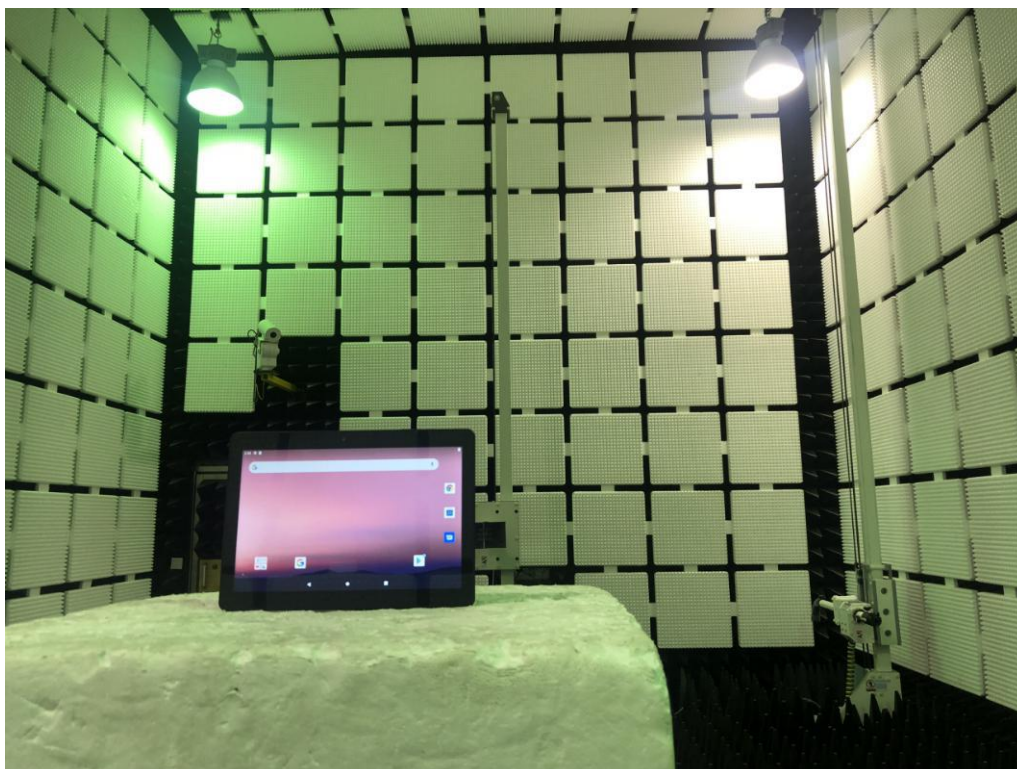
Fig. 2 (Above 1GHz)
