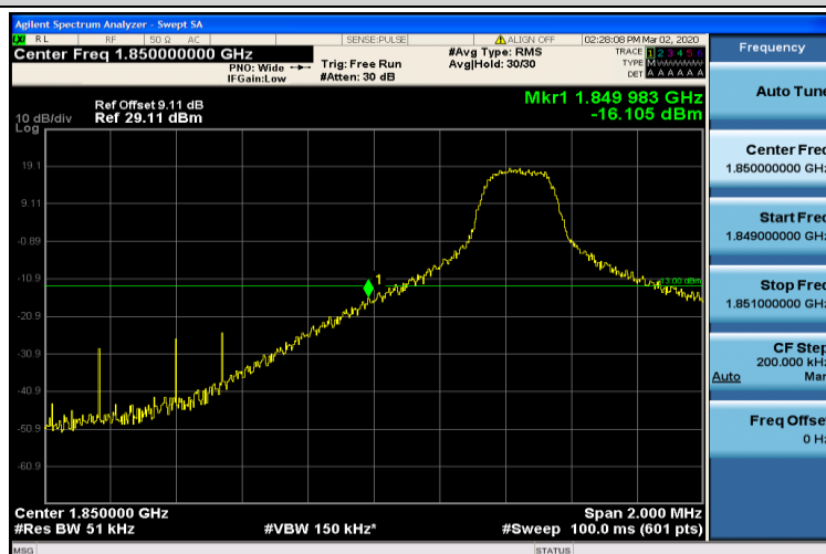
Band2-5MHz-16QAM-18625-1RB#0
