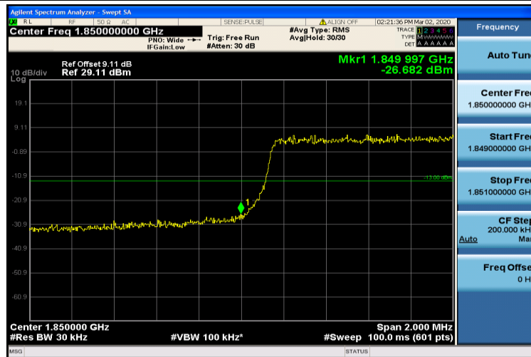
Band2-3MHz-QPSK-18615-15RB#0
