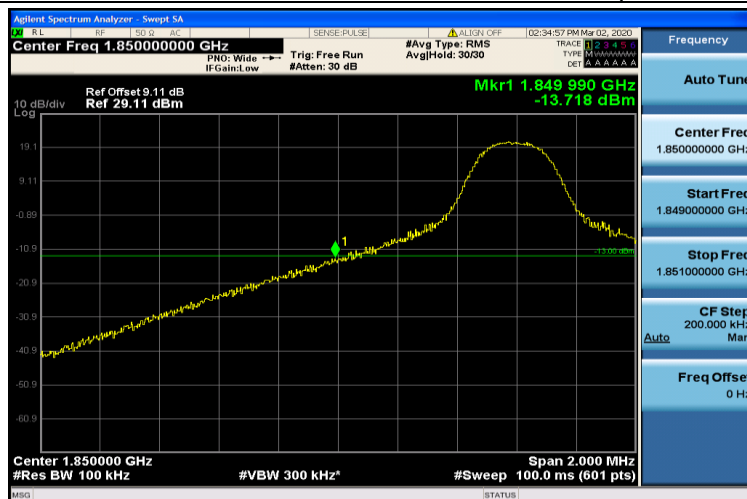
Band2-10MHz-QPSK-18650-1RB#0
