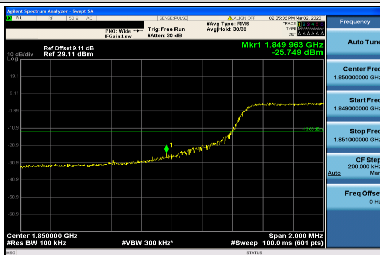
Band2-10MHz-QPSK-18650-50RB#0
