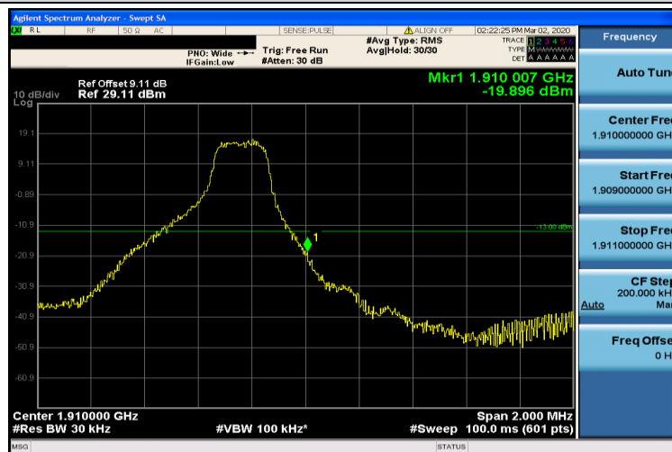
Band2-3MHz-QPSK-19185-15RB#14
