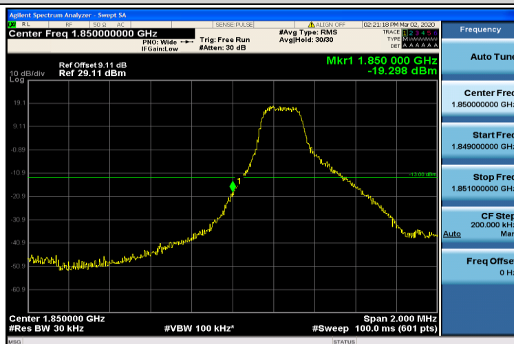
Band2-3MHz-QPSK-18615-1RB#0
