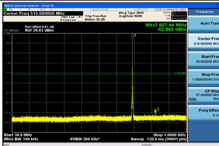
Band12-1.4MHz-QPSK-23017-1RB#0-30~1000MHz
