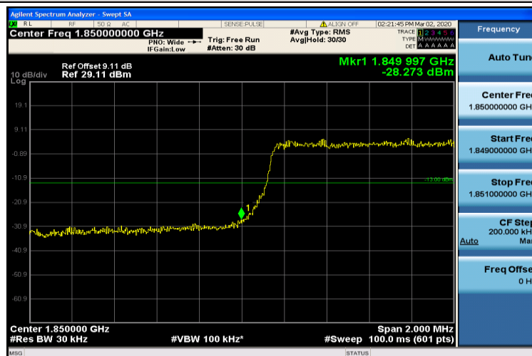
Band2-3MHz-16QAM-18615-15RB#0
