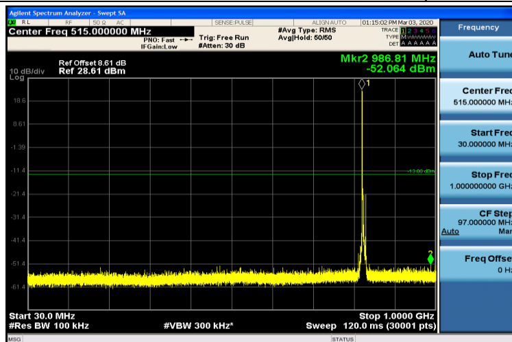
Band5-5MHz-QPSK-20425-1RB#0-30~1000MHz
