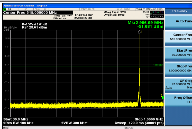
Band5-3MHz-QPSK-20635-1RB#0-30~1000MHz
