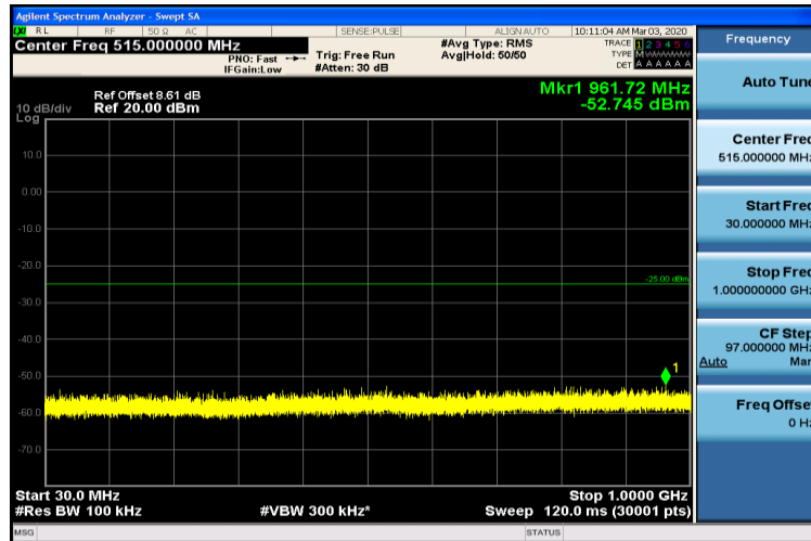
Band7-20MHz-QPSK-20850-1RB#0-30~1000MHz
