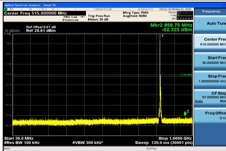
Band5-3MHz-QPSK-20415-1RB#0-30~1000MHz
