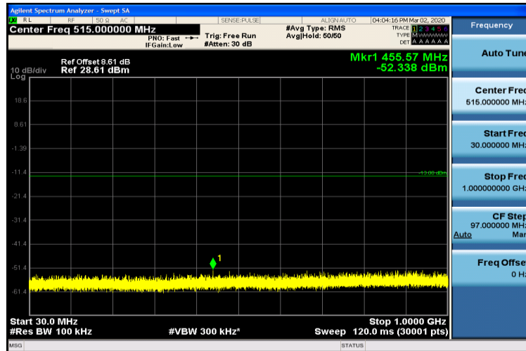
Band4-10MHz-QPSK-20000-1RB#0-30~1000MHz
