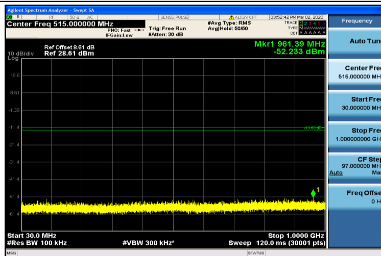
Band4-1.4MHz-QPSK-20393-1RB#0-30~1000MHz
