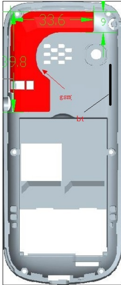
c. Antenna
