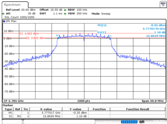
a_5785MHz_Chain 0 15.866MHz
