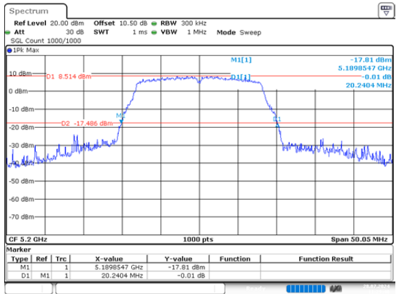
a_5200MHz_Chain 0 20.240MHz
