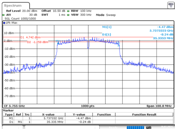
n40_5755MHz_Chain 0 35.335MHz
