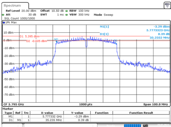
n40_5795MHz_Chain 1 35.235MHz
