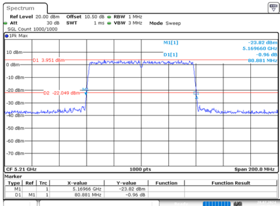
ac80_5210MHz_Chain 0 80.881MHz
