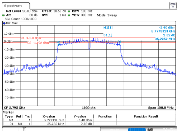
n40_5795MHz_Chain 0 35.235MHz
