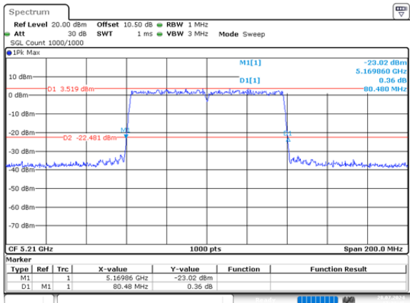
ac80_5210MHz_Chain 1 80.480MHz
