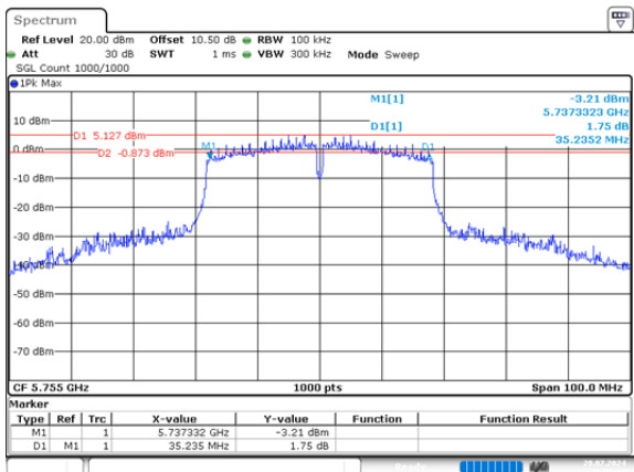
n40_5755MHz_Chain 1 35.235MHz
