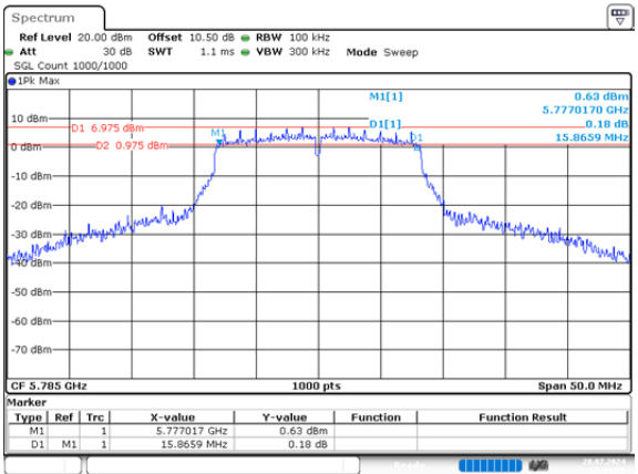
a_5785MHz_Chain 1 15.866MHz
