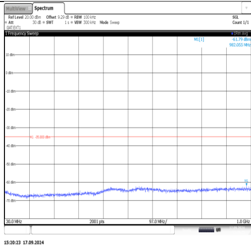
Band38-20MHz-QPSK-38150-1RB#0-20000-PASS
