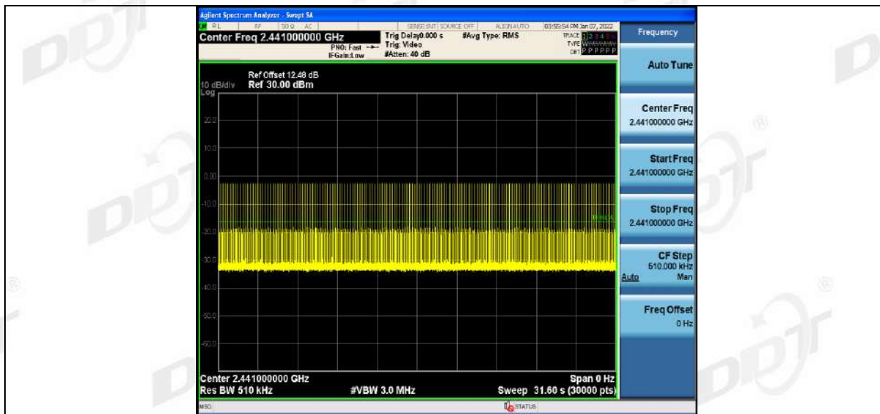
2DH5_Ant1_Hop
