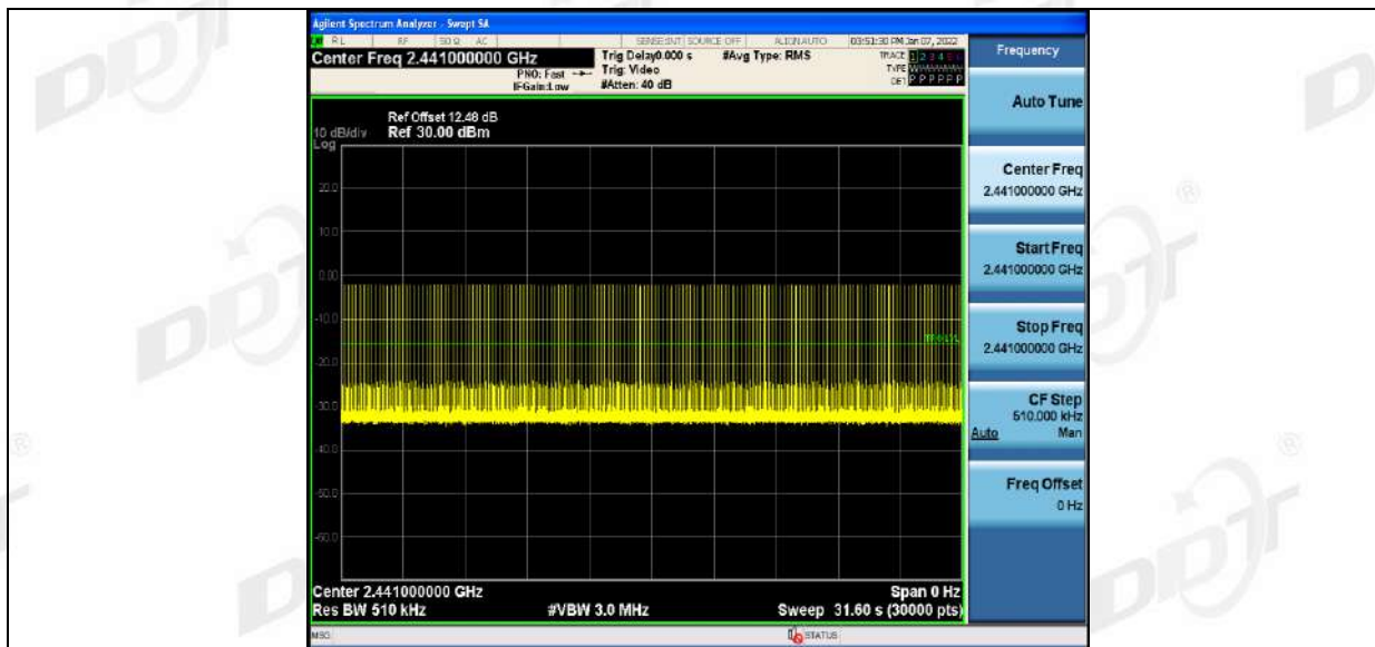
DH5_Ant1_Hop
