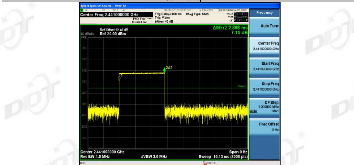
DH5_Ant1_Hop
