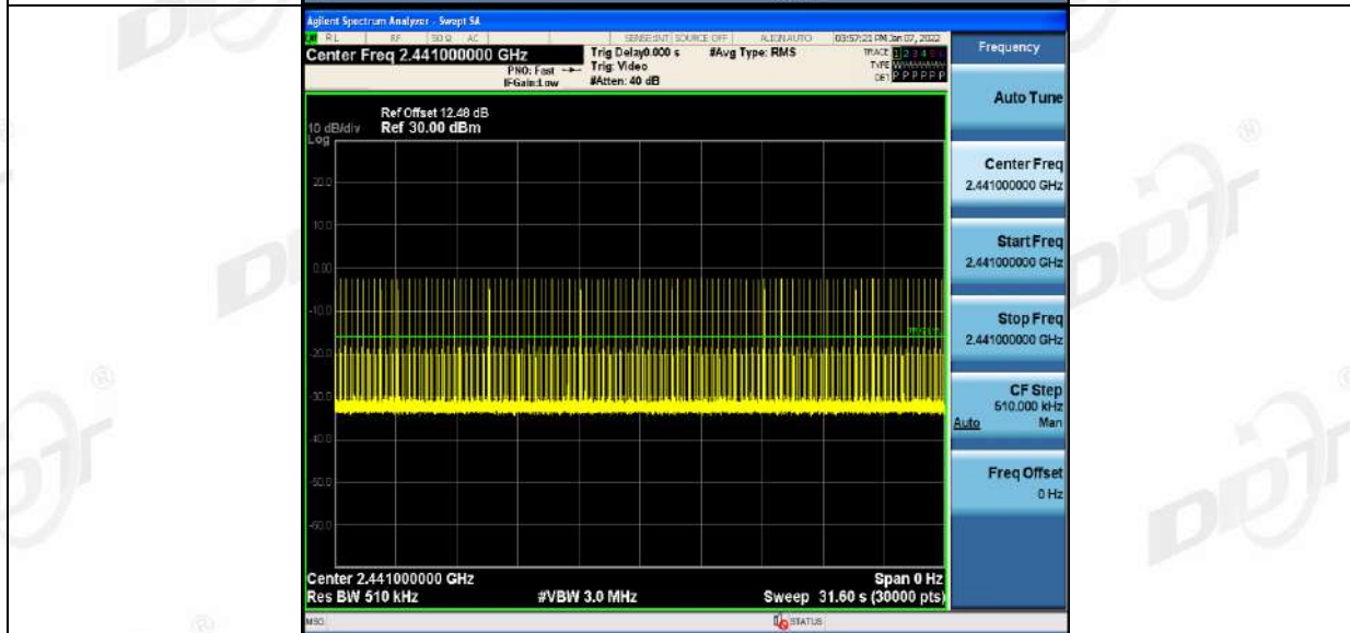
3DH1_Ant1_Hop
