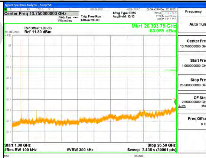
BLE BT4.0 Ant1 2442 0~Reference
