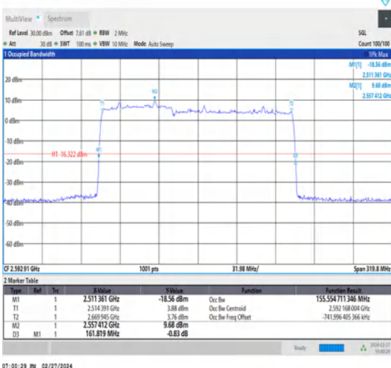
NTNV_CA_n41C_PC3_30+30_60+100_M+M_Ant1_TID5 _1_#1
