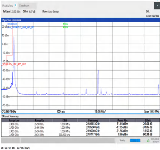
NTNV_CA_n41C_PC3_30+30_80+60_L+L_TID1_1_#1
