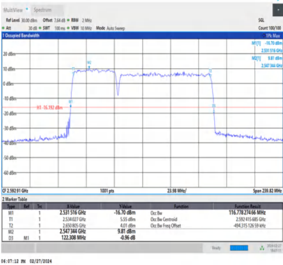
NTNV_CA_n41C_PC3_30+30_40+80_M+M_Ant1_TID7_1_#1
