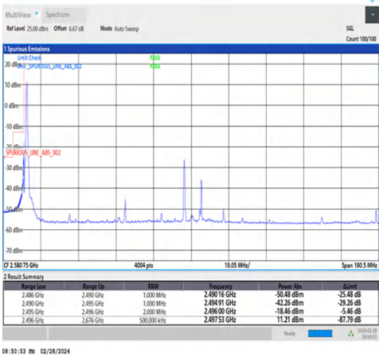
NTNV_CA_n41C_PC3_30+30_80+100_L+L_TID4_1_#1
