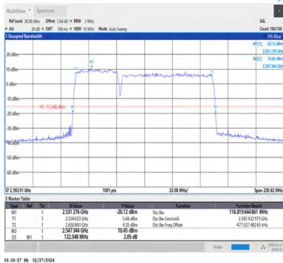
NTNV_CA_n41C_PC3_30+30_40+80_M+M_Ant1_TID6_1_#1
