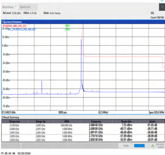
NTNV_CA_n41C_PC3_30+30_80+80_H+H_TID5_1_#1
