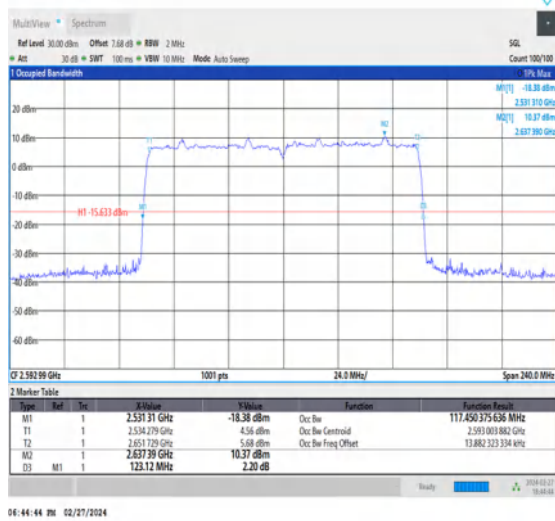
NTNV_CA_n41C_PC3_30+30_60+60_M+M_Ant1_TID5_1_#1
