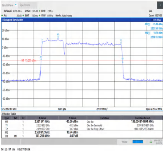
NTNV_CA_n41C_PC3_30+30_40+100_M+M_Ant1_TID8 _1_#1
