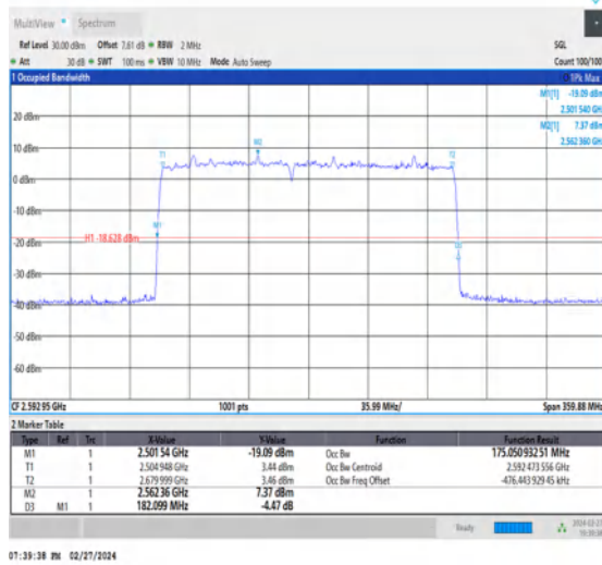
NTNV_CA_n41C_PC3_30+30_80+100_M+M_Ant1_TID9_1_#1
