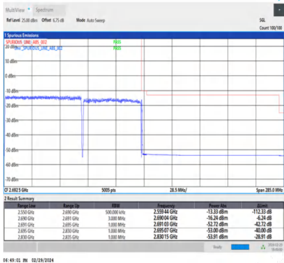
NTNV_CA_n41C_PC3_30+30_80+60_H+H_TID3_1_#1
