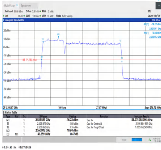
NTNV_CA_n41C_PC3_30+30_40+100_M+M_Ant1_TID3_1_#1
