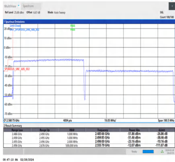
NTNV_CA_n41C_PC3_30+30_80+100_L+L_TID3_1_#1
