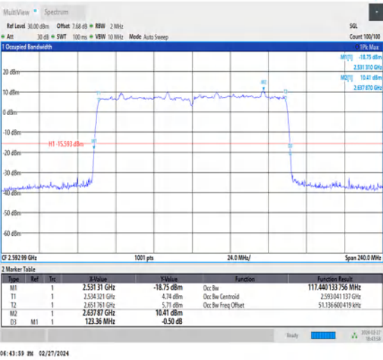
NTNV_CA_n41C_PC3_30+30_60+60_M+M_Ant1_TID2_1_#1
