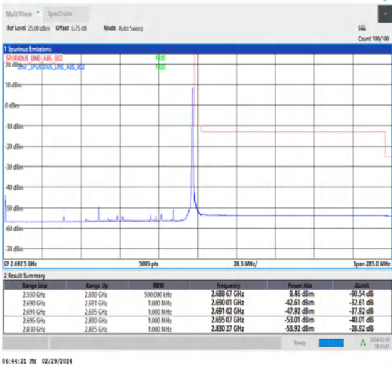
NTNV_CA_n41C_PC3_30+30_80+60_H+H_TID2_1_#1
