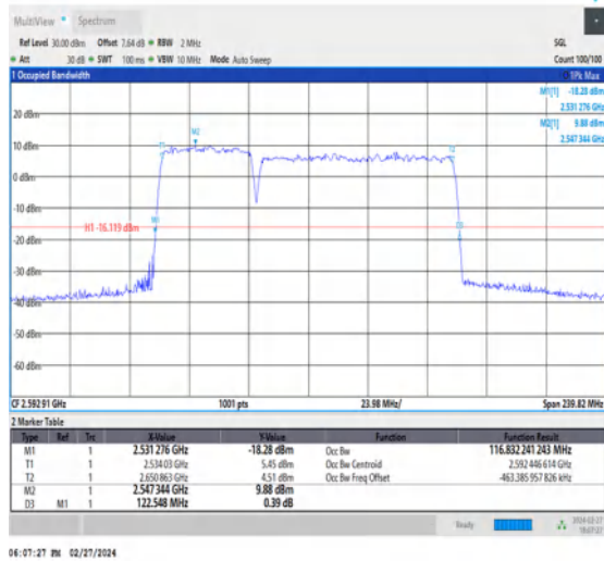
NTNV_CA_n41C_PC3_30+30_40+80_M+M_Ant1_TID8_1_#1
