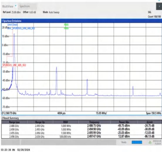
NTNV_CA_n41C_PC3_30+30_40+100_L+L_TID1_1_#1
