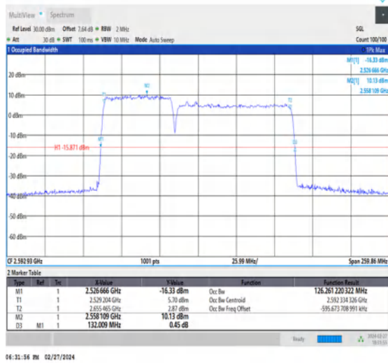
NTNV_CA_n41C_PC3_30+30_50+80_M+M_Ant1_TID7_1_#1
