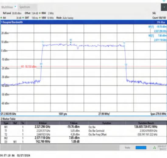
NTNV_CA_n41C_PC3_30+30_60+80_M+M_Ant1_TID7_1_#1
