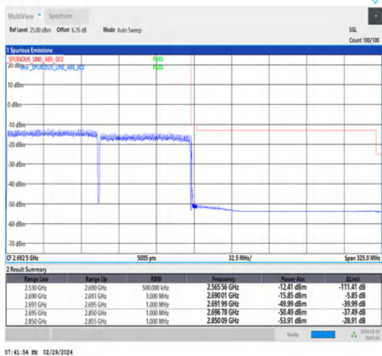
NTNV_CA_n41C_PC3_30+30_80+80_H+H_TID6_1_#1
