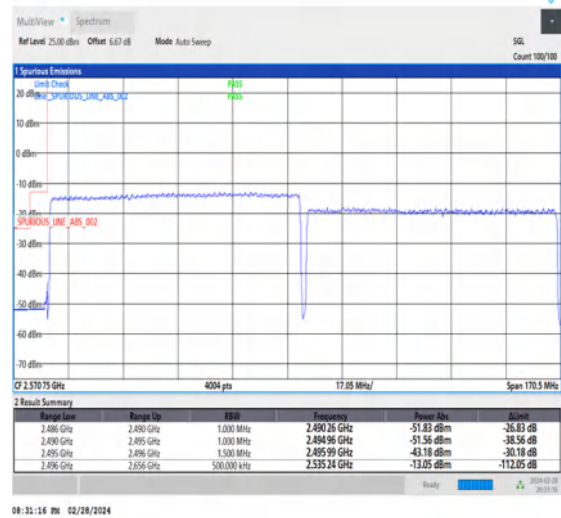
NTNV_CA_n41C_PC3_30+30_80+80_L+L_TID3_1_#1
