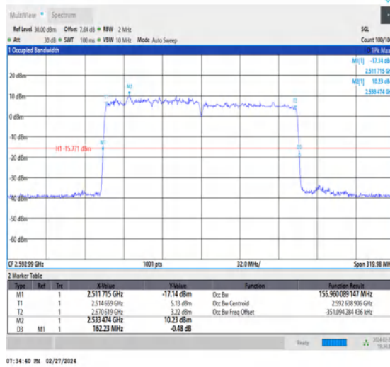
NTNV_CA_n41C_PC3_30+30_80+80_M+M_Ant1_TID4_1_#1
