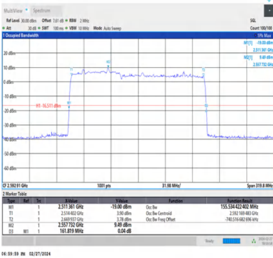
NTNV_CA_n41C_PC3_30+30_60+100_M+M_Ant1_TID3 _1_#1
