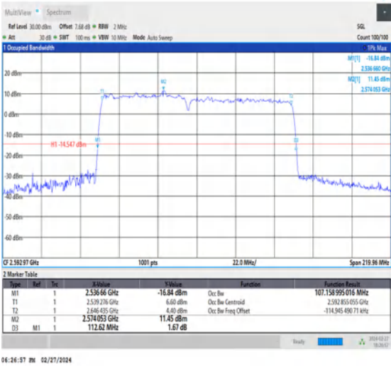
NTNV_CA_n41C_PC3_30+30_50+60_M+M_Ant1_TID7_1_#1
