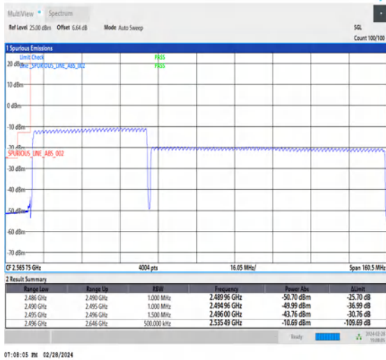
NTNV_CA_n41C_PC3_30+30_50+100_L+L_TID6_1_#1
