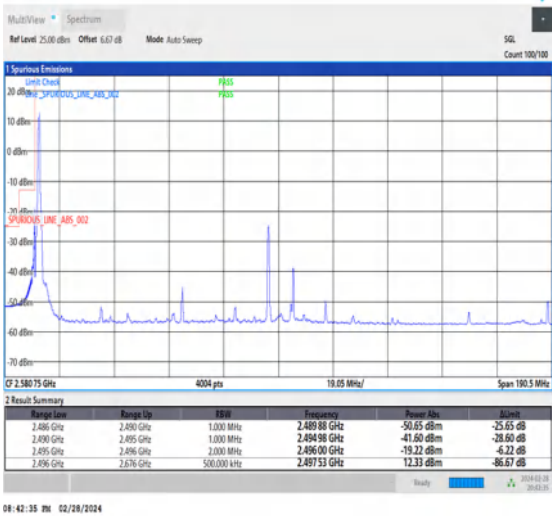
NTNV_CA_n41C_PC3_30+30_80+100_L+L_TID1_1_#1
