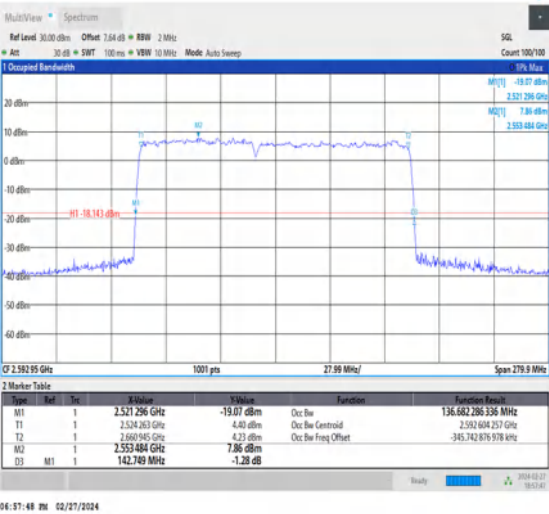
NTNV_CA_n41C_PC3_30+30_60+80_M+M_Ant1_TID9_1_#1
