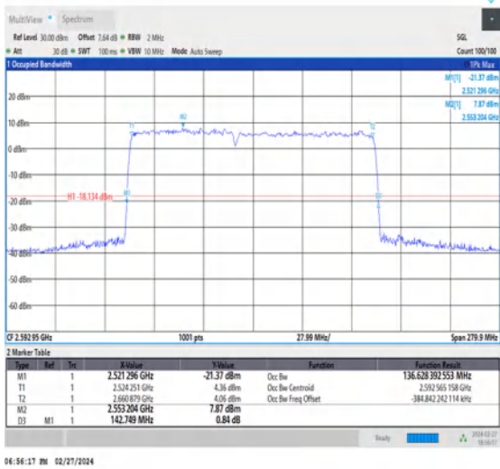
NTNV_CA_n41C_PC3_30+30_60+80_M+M_Ant1_TID3_1_#1
