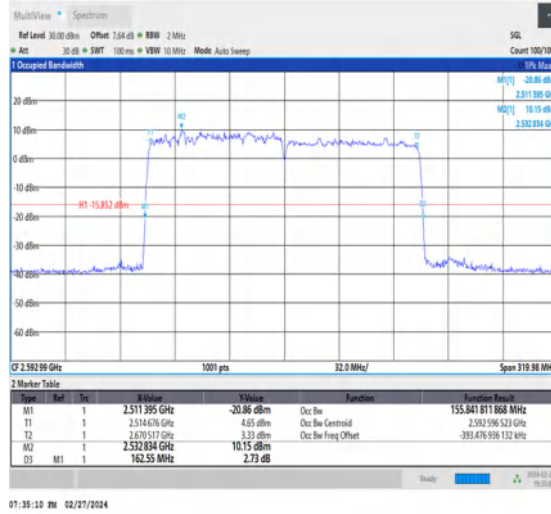
NTNV_CA_n41C_PC3_30+30_80+80_M+M_Ant1_TID6_1_#1
