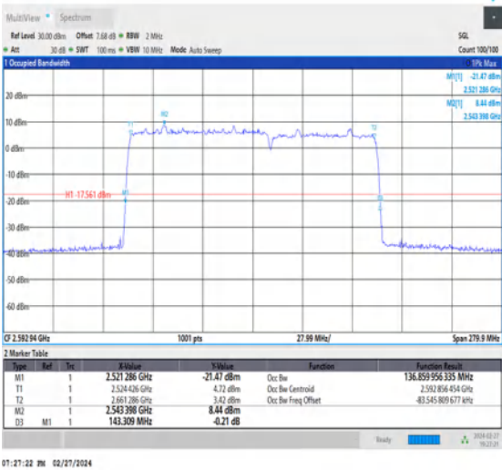
NTNV_CA_n41C_PC3_30+30_80+60_M+M_Ant1_TID3_1_#1
