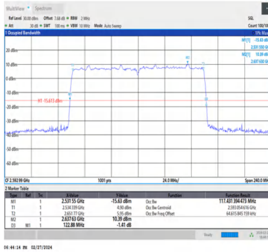
NTNV_CA_n41C_PC3_30+30_60+60_M+M_Ant1_TID3_1_#1
