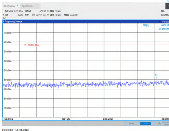
Band66-20MHz-QPSK-132072-1RB#0-Range2:0.15~30MHz
