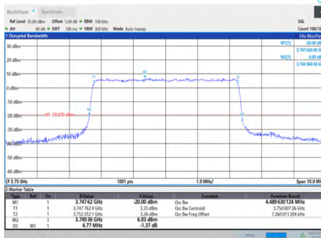
Band43-5MHz-QPSK-45090-25RB#0
