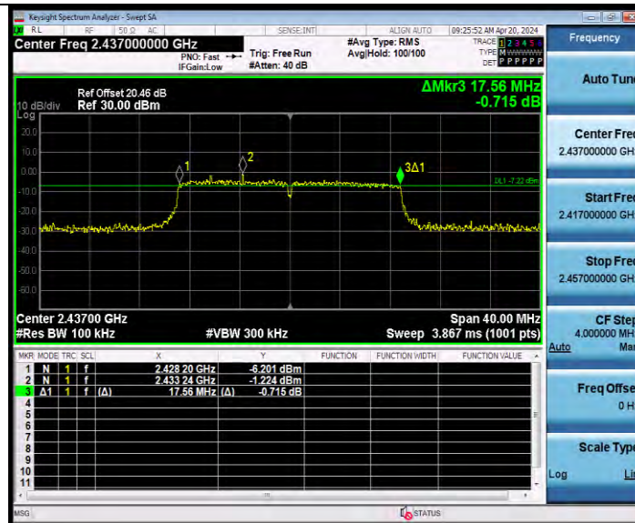
11N20MIMO Ant9 2437
