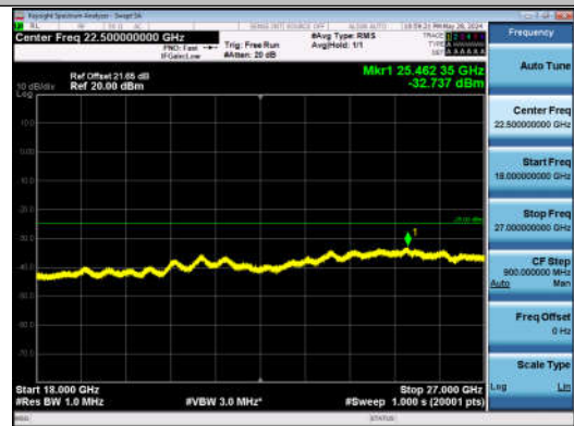
7-7-20MHz-20MHz-QPSK-QPSK-20850-21048-1RB#0-0RB #0-18000~27000MHz-PASS
