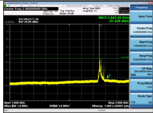
7-7-20MHz-20MHz-QPSK-QPSK-20850-21048-1RB#0-0RB #0-1000~3000MHz-PASS
