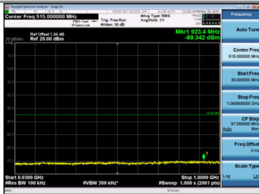
7-7-20MHz-20MHz-QPSK-QPSK-21001-21199-1RB#0-0R B#0-30~1000MHz-PASS
