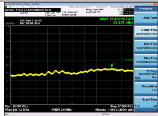
41-41-20MHz-20MHz-QPSK-QPSK-40340-40538-1RB#0-0 RB#0-18000~27000MHz-PASS
