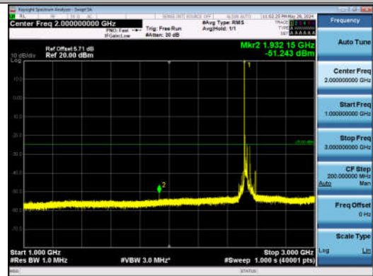
7-7-20MHz-20MHz-QPSK-QPSK-21001-21199-1RB#0-0RB #0-1000~3000MHz-PASS
