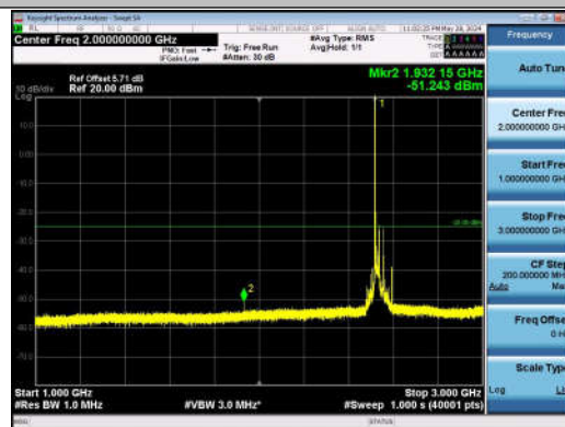
7-7-20MHz-20MHz-QPSK-QPSK-21001-21199-1RB#0-0RB #0-1000~3000MHz-PASS
