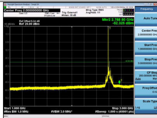
41-41-20MHz-20MHz-QPSK-QPSK-40641-40839-1RB#0-0 RB#0-1000~3000MHz-PASS
