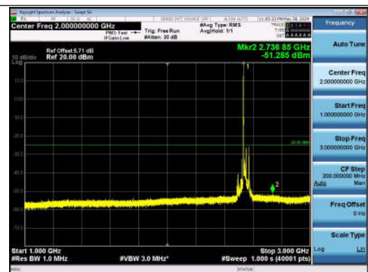
7-7-20MHz-20MHz-QPSK-QPSK-21152-21350-1RB#0-0RB #0-1000~3000MHz-PASS
