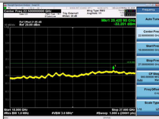
41-41-20MHz-20MHz-QPSK-QPSK-40340-40538-1RB#0-0 RB#0-18000~27000MHz-PASS
