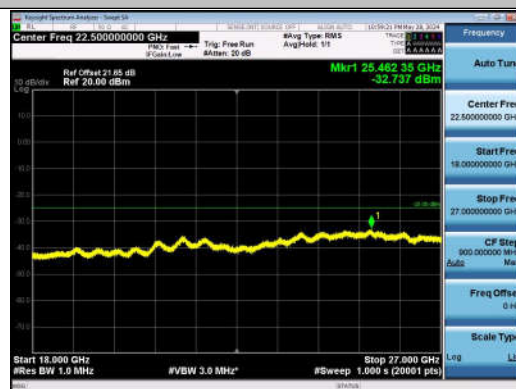
7-7-20MHz-20MHz-QPSK-QPSK-20850-21048-1RB#0-0RB #0-18000~27000MHz-PASS
