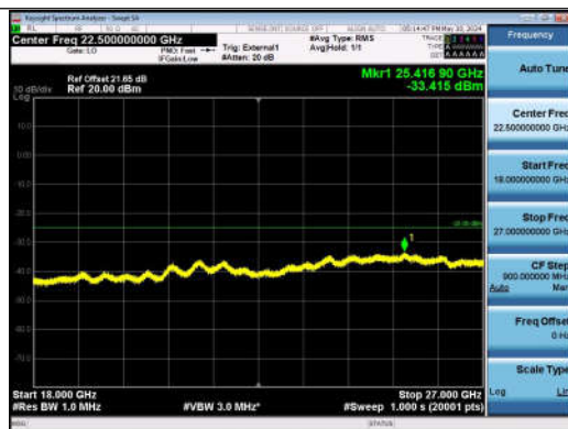
41-41-20MHz-20MHz-QPSK-QPSK-40641-40839-1RB#0-0 RB#0-18000~27000MHz-PASS
