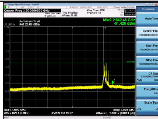
7-7-20MHz-20MHz-QPSK-QPSK-20850-21048-1RB#0-0RB #0-1000~3000MHz-PASS
