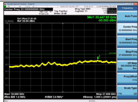
7-7-20MHz-20MHz-QPSK-QPSK-21152-21350-1RB#0-0RB #0-18000~27000MHz-PASS
