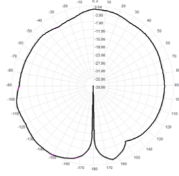
2400.0MHz Total(E2-YZ), Max= 0.02dBi
