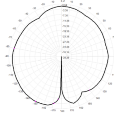
2440.0MHz Total(E2-YZ), Max= 0.10dBi
