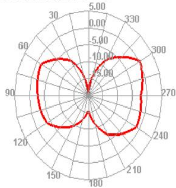
490.000MHz E2
