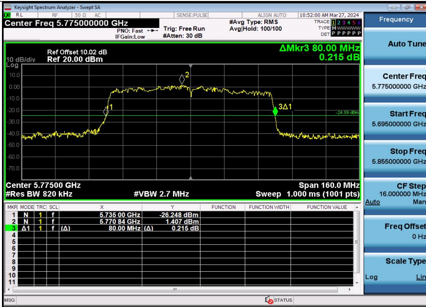
11AC80SISO-Ant2-5775
