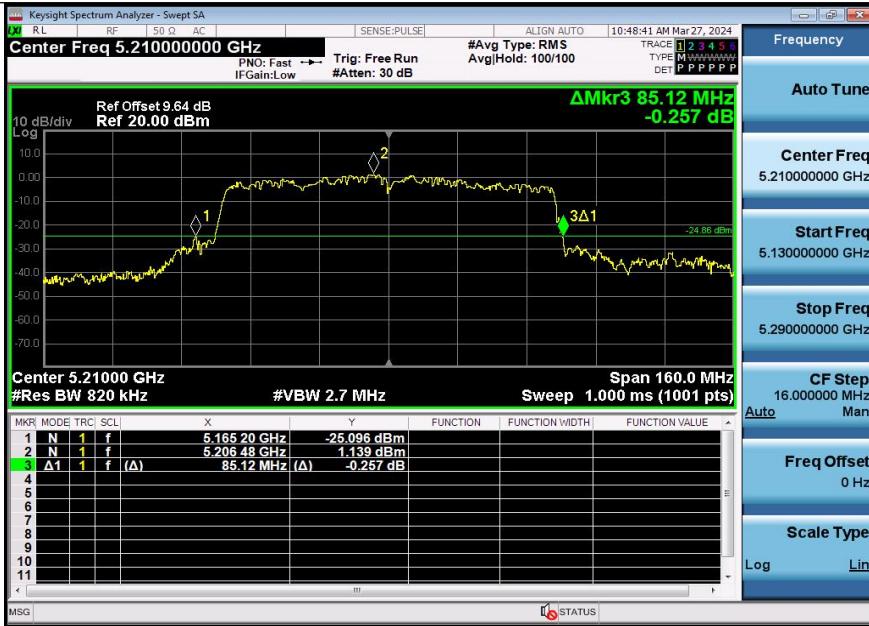
11AC80SISO-Ant2-5210
