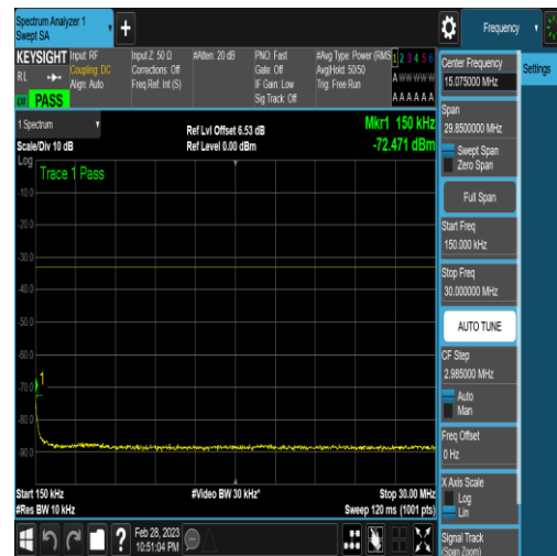
NTNV_N78-3700-3800_PC2_30_20_H_TID16_N/ A_0.15_30_#1
