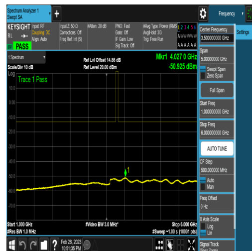
NTNV_N78-3700-3800_PC2_30_20_H_TID16_N/ A_1000_6000_#1
