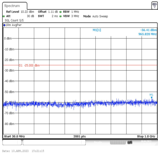
41-41-5MHz-20MHz-QPSK-QPSK-41373-41490-1RB#0-0RB#0-30~1000MHz
