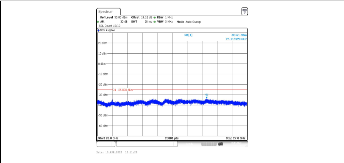
20MHz-20MHz-37901-38099
