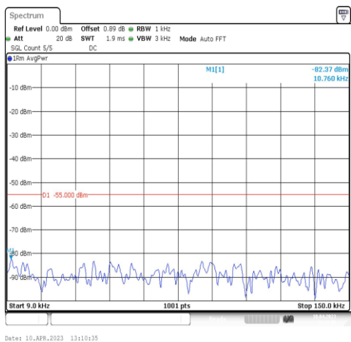
20MHz-20MHz-37901-38099
