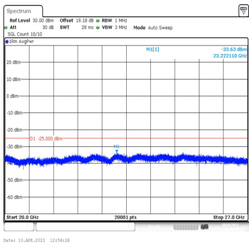
20MHz-20MHz-37850-38048
