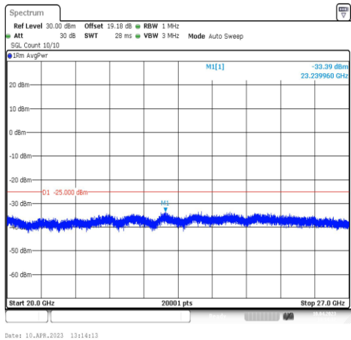
20MHz-20MHz-37901-38099
