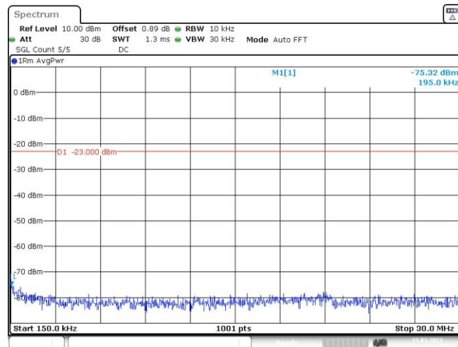
Band12-1.4MHz-QPSK-23017-1RB#0-Range2:0.15~30MHz
