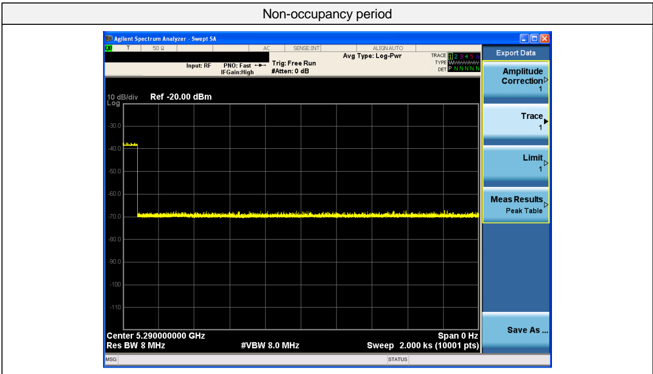
80MHz/5290MHz
