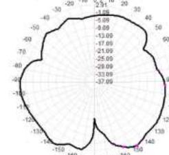
2400.0MHz Total(E2-YZ), Max= 2.91dBi
