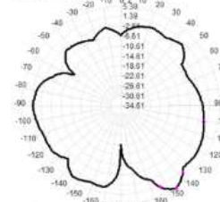
2500.0MHz Total(E2-YZ), Max= 5.39dBi
