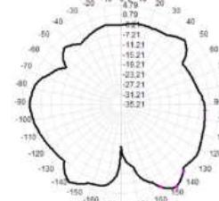
2450.0MHz Total(E2-YZ), Max= 4.79dBi
