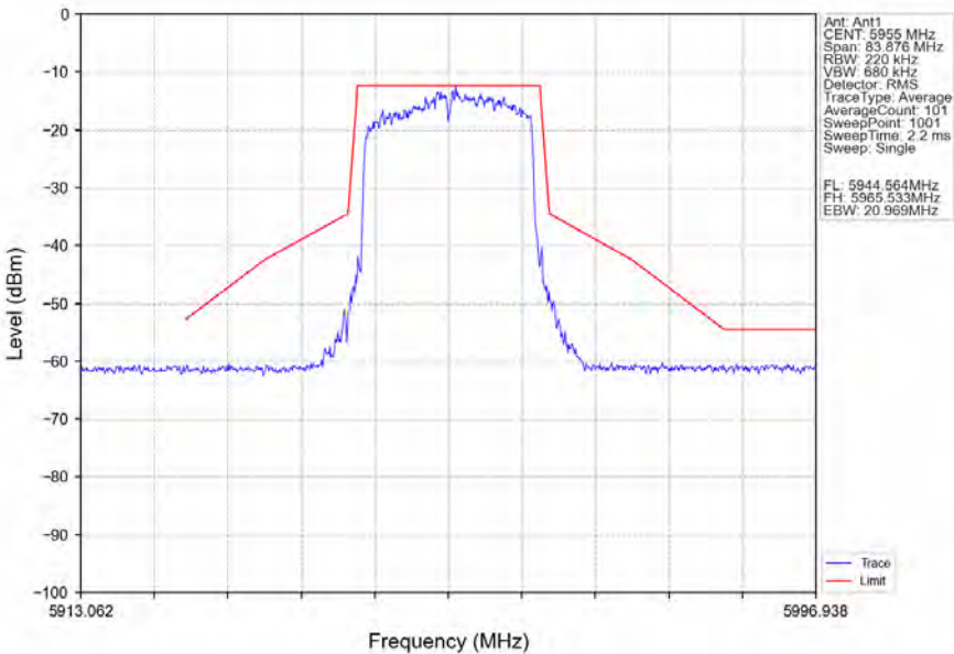
802.11ax(HEW20)_LCH_5955MHz_RU242_Left_Ant1_NTNV
