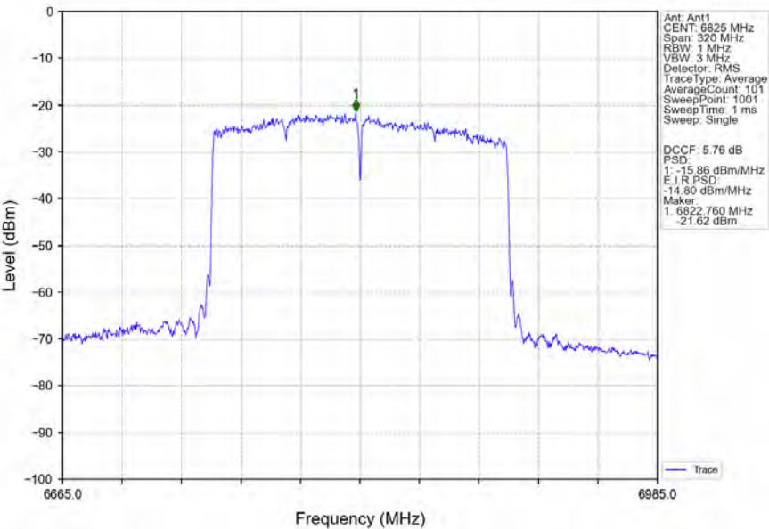
802.11ax(HEW160)_HCH_6825MHz_2xRU996_Left_Ant1_NTNV
