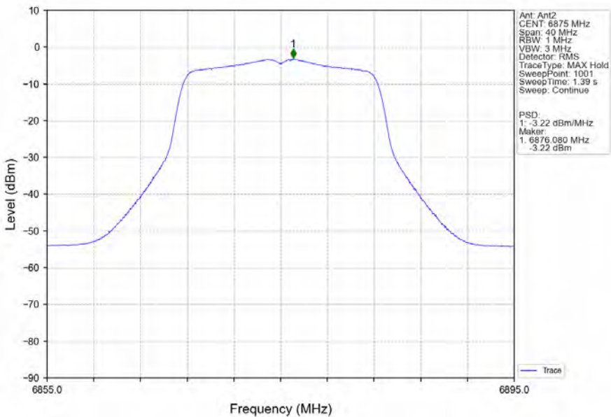
802.11a_HCH_6875MHz_Ant2_NTNV
