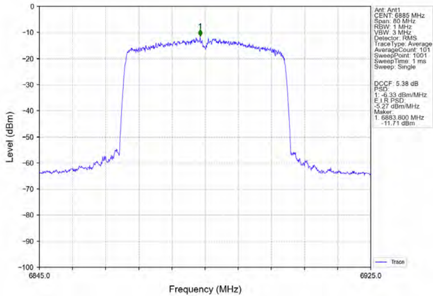
802.11ax(HEW40)_HCH_6885MHz_RU484_Left_Ant1_NTNV
