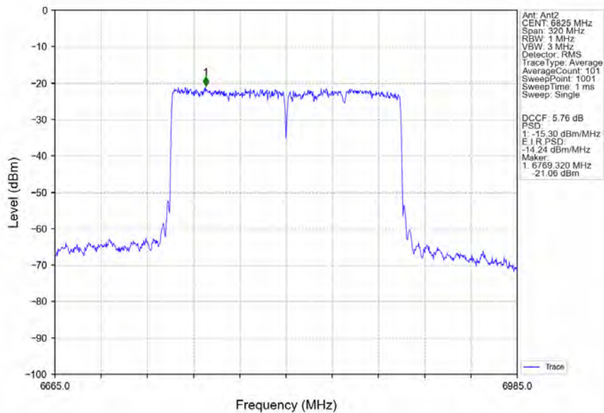
802.11ax(HEW160)_HCH_6825MHz_2xRU996_Left_Ant2_NTNV
