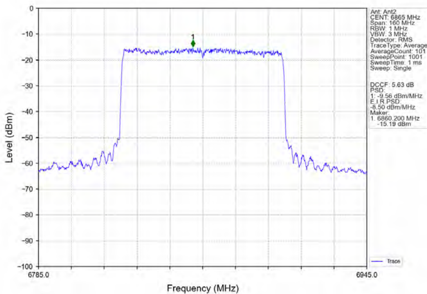
802.11ax(HEW80)_HCH_6865MHz_RU996_Left_Ant2_NTNV
