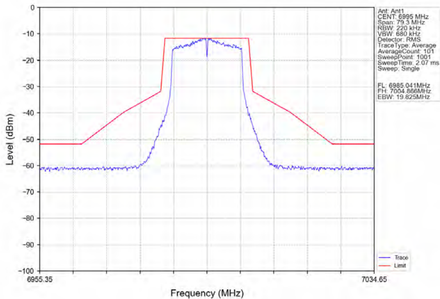
802.11a_MCH_6995MHz_Ant1_NTNV
