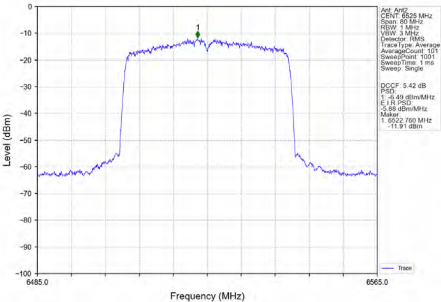
802.11ax(HEW40)_HCH_6525MHz_RU484_Left_Ant2_NTNV
