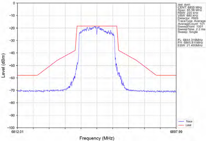
802.11ax(HEW20)_HCH_6855MHz_RU242_Left_Ant1_NTNV
