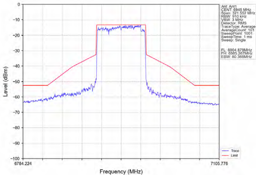
802.11ax(HEW80)_LCH_6945MHz_RU996_Left_Ant1_NTNV
