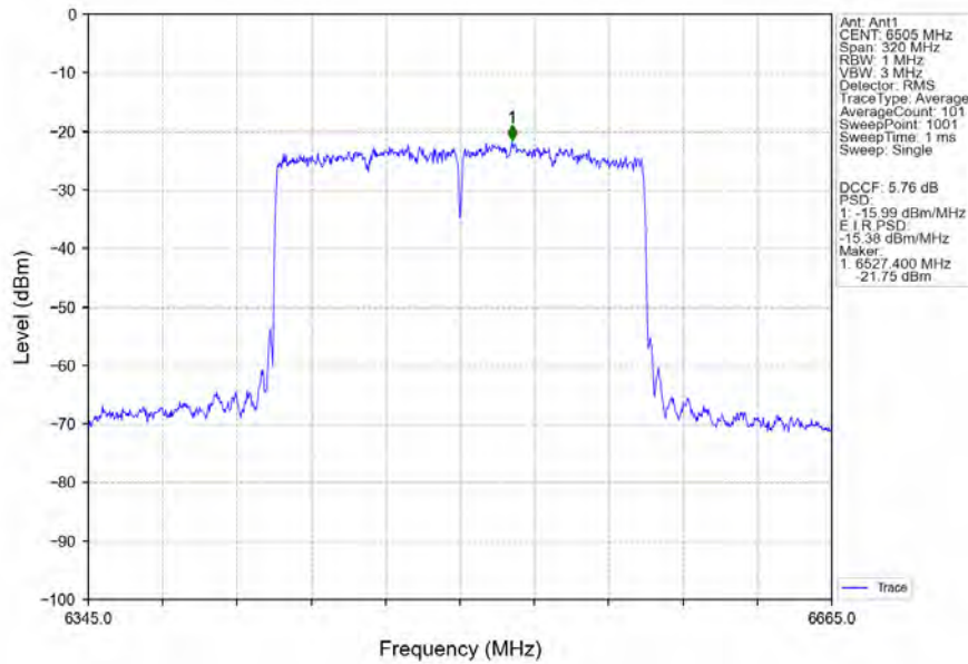
802.11ax(HEW160)_HCH_6505MHz_2xRU996_Left_Ant1_NTNV
