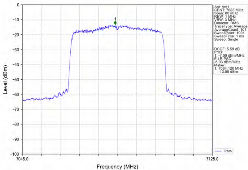
802.11ax(HEW40)_HCH_7085MHz_RU484_Left_Ant1_NTNV
