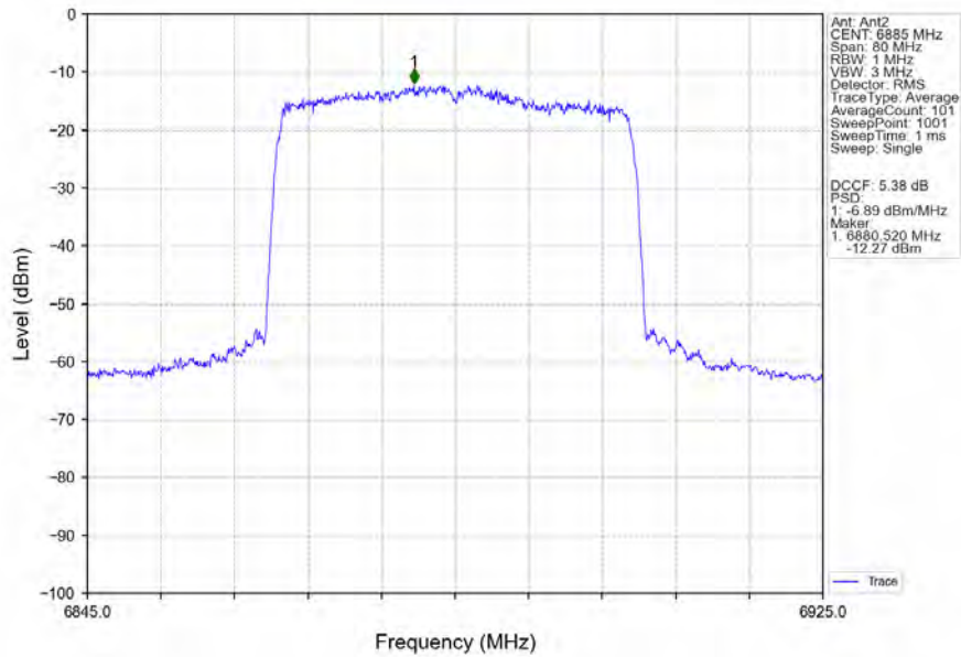
802.11ax(HEW40)_HCH_6885MHz_RU484_Left_Ant2_NTNV
