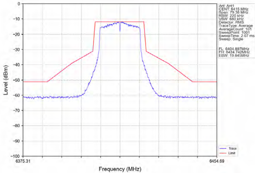
802.11a_HCH_6415MHz_Ant1_NTNV
