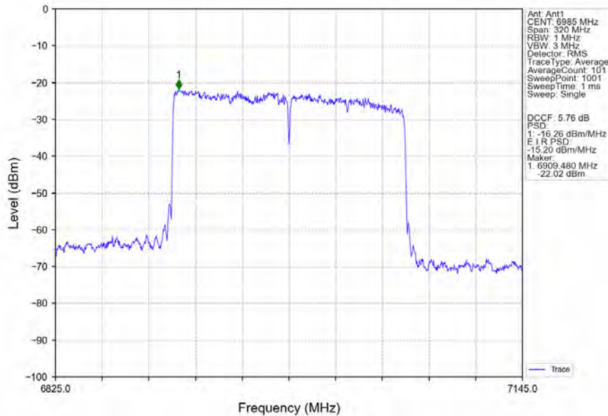
802.11ax(HEW160)_MCH_6985MHz_2xRU996_Left_Ant1_NTNV
