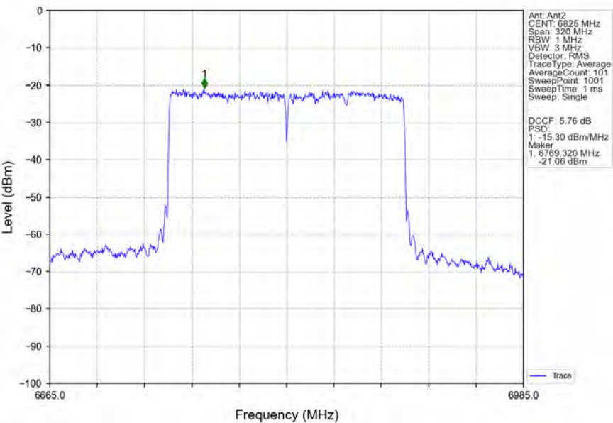
802.11ax(HEW160)_HCH_6825MHz_2xRU996_Left_Ant2_NTNV
