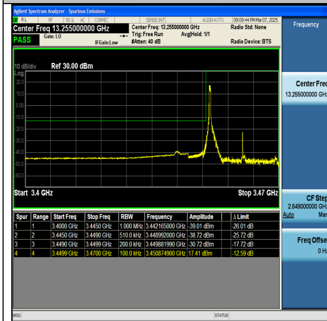
NTNV-n77(3450-3550)-PC2-30-20-L-CP-QPSK- Edge_1RB_Left-PASS
