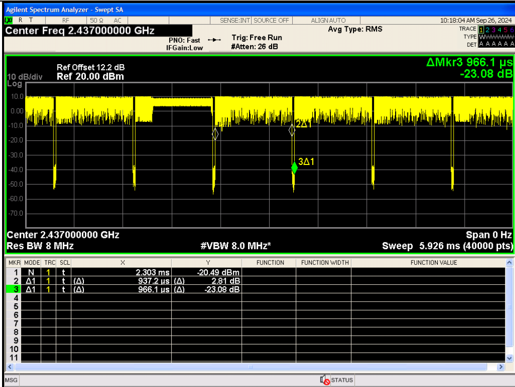
IEEE 802.11b_20MHz_Channel 6
