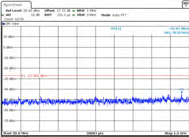
11AC80SISO-Ant1-5775-30~1000-PASS
