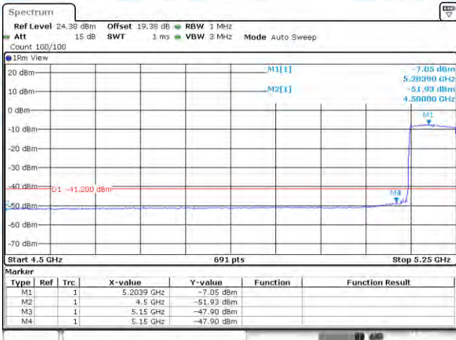
11AX80SISO-Ant1-5210-PASS
