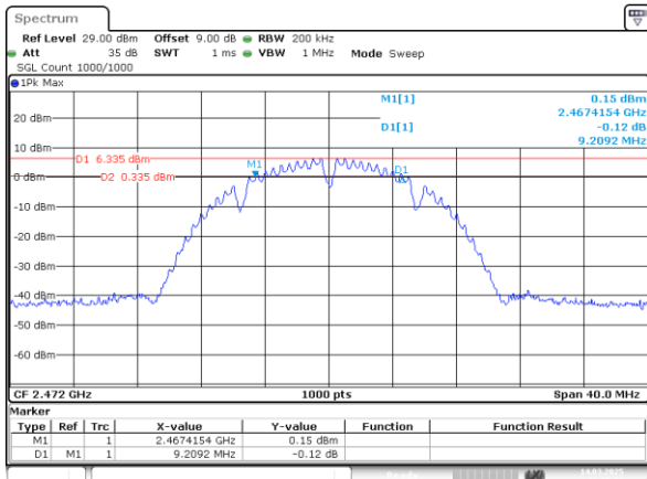
802.11b_2472MHz
