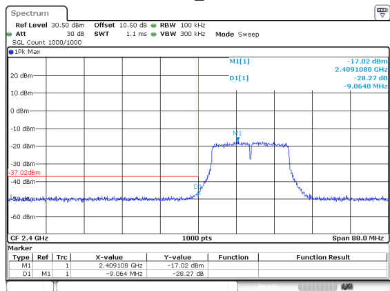
802.11n20_2412MHz
