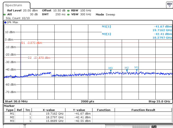
802.11b_2472MHz
