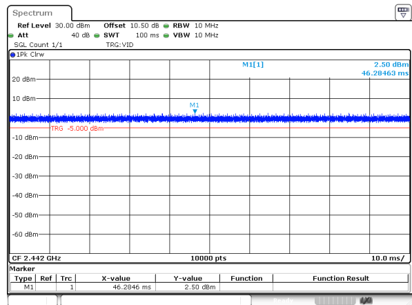
802.11n20_2442MHz
