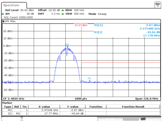
802.11b_2472MHz
