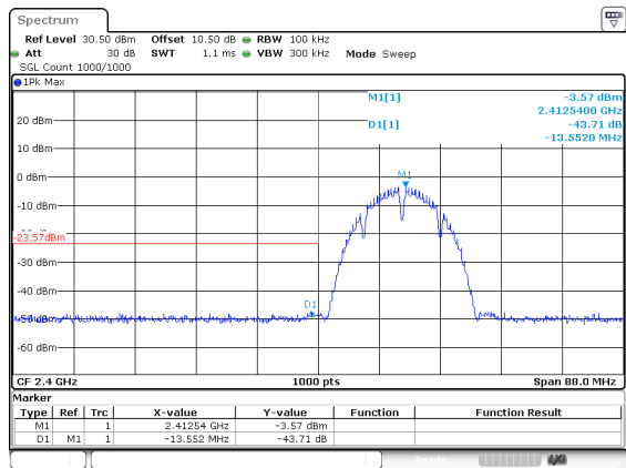
802.11b_2412MHz
