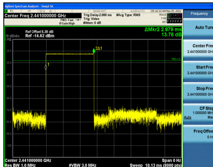
2DH1_Ant1_Hop
