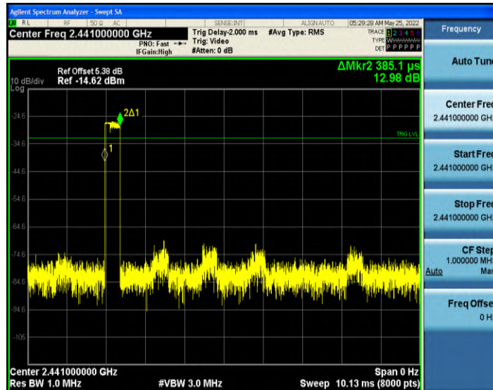
2DH3_Ant1_Hop
