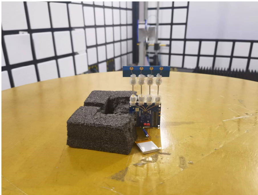
Antenna Mode 2 Stand
