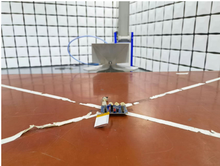
1GHz-18GHz Vertical
