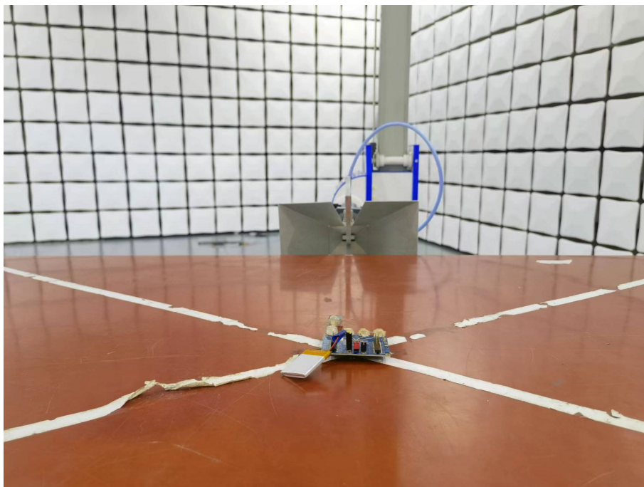
1GHz-18GHz Horizontal
