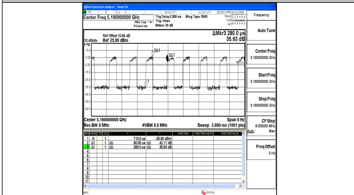
NTNV-11N40MIMO-Ant1-5190
